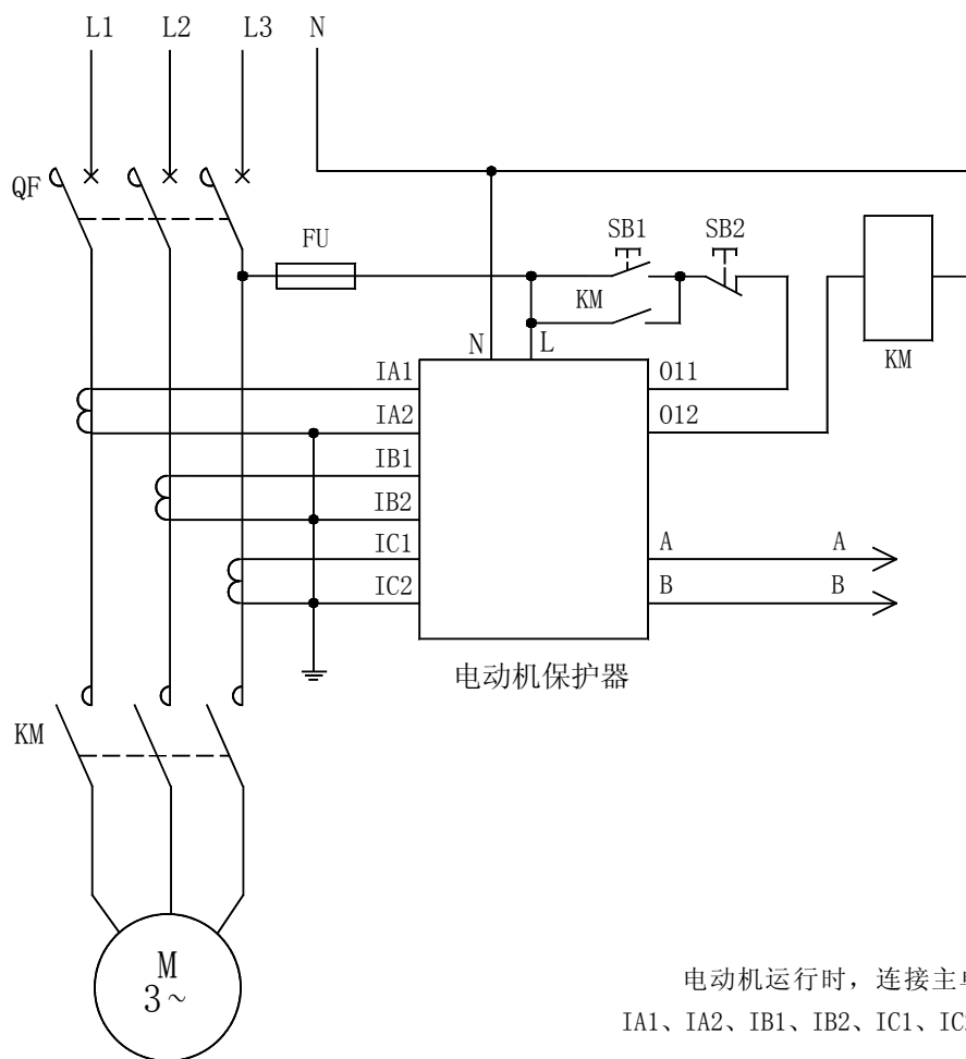
AMDGH-X/E32□ 系列电动机保护器应用电气原理图
