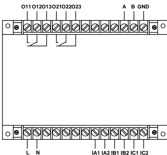
AMDGH-X/E322 系列保护器主单元接线端子图
