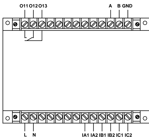
AMDGH-X/E321 系列保护器主单元接线端子图
