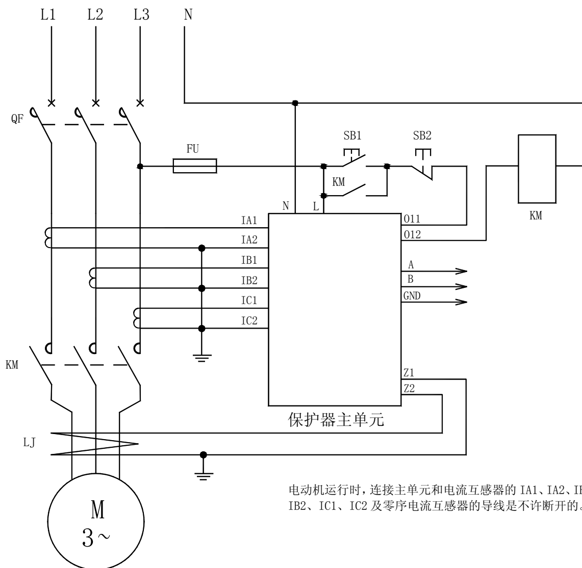
AMDGH-X/E31□ 系列电动机保护器应用电气原理图
