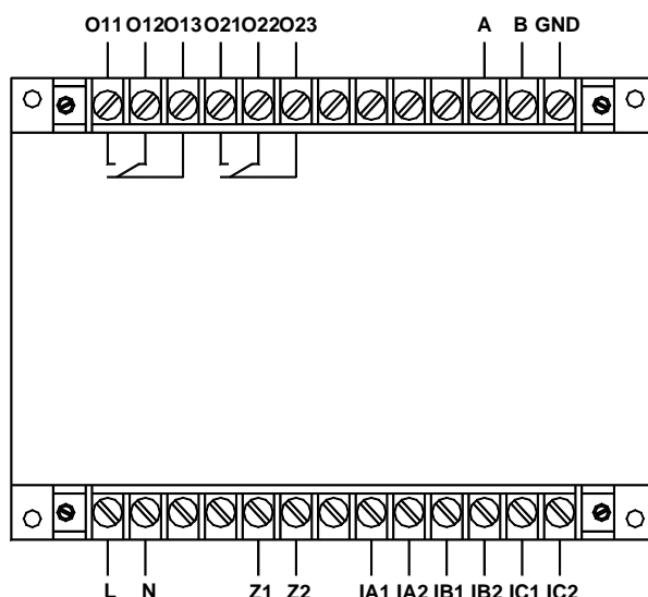
AMDGH-X/E312 系列保护器主单元接线端子图
