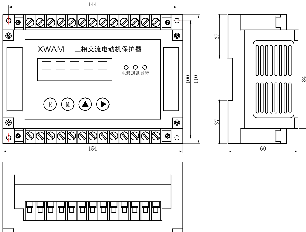
AMDGH-X/E31□ 系列电动机保护器主单元外形及安装孔尺寸
