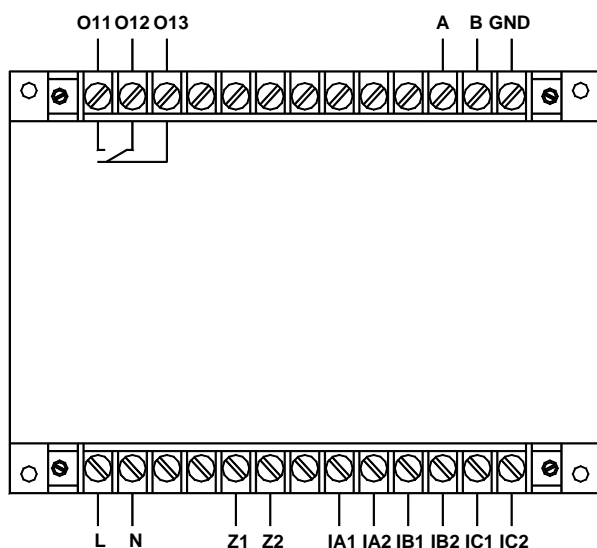
AMDGH-X/E311 系列保护器主单元接线端子图
