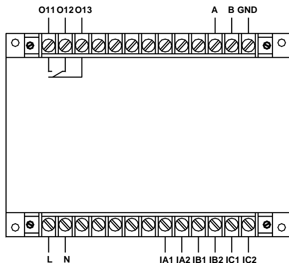
AMDGH-X/E301 系列保护器主单元接线端子图
