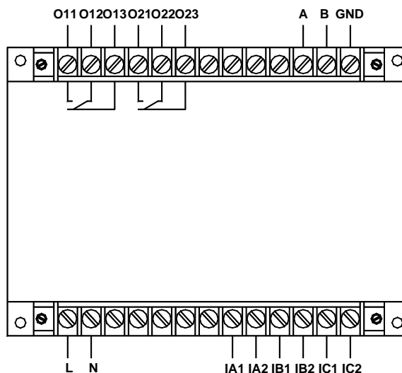
AMDGH-X/E302 系列保护器主单元接线端子图
