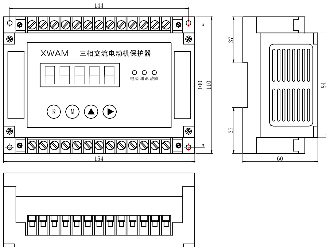
AMDGH-X/E30□ 系列电动机保护器主单元外形及安装孔尺寸
