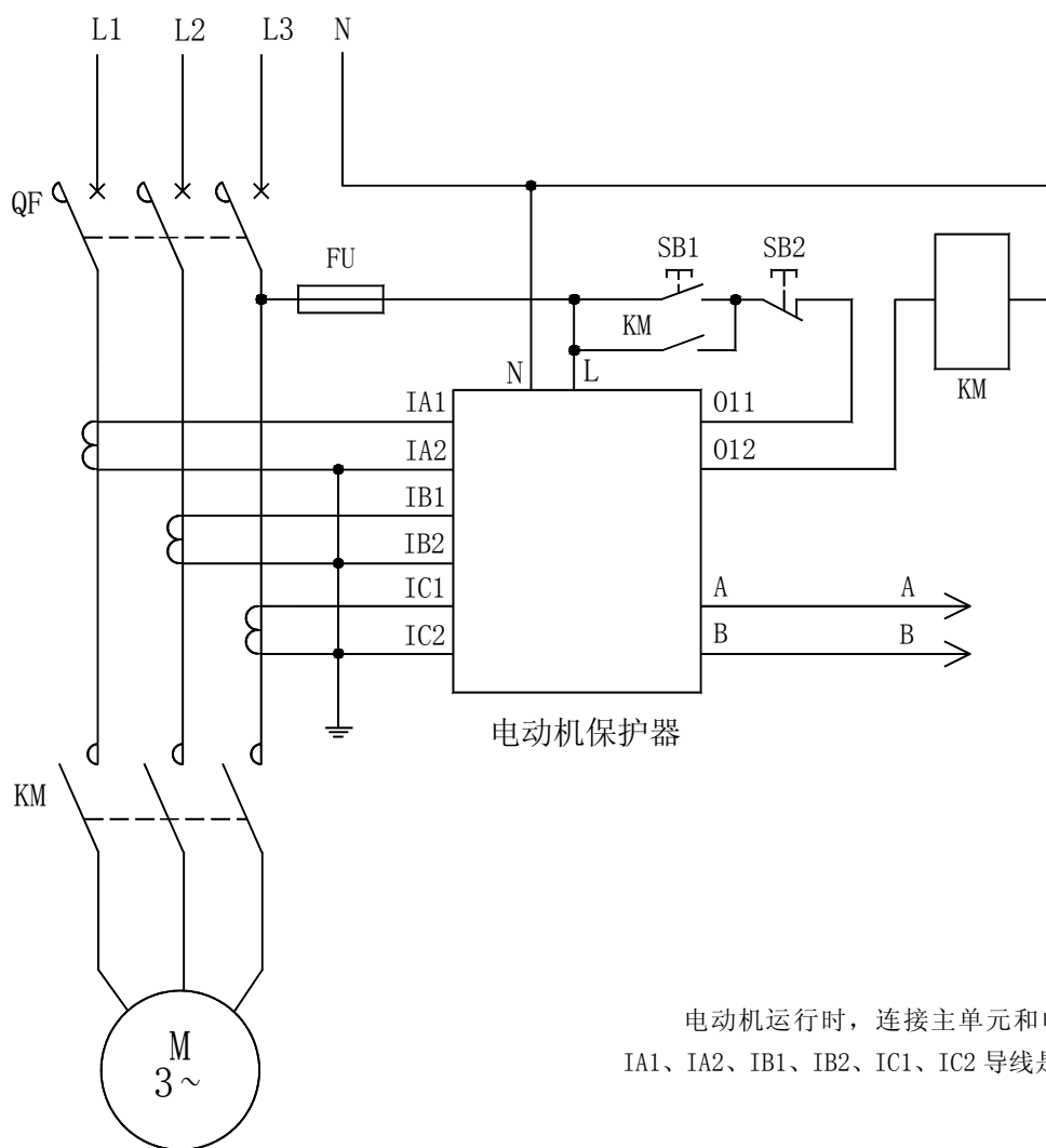
AMDGH-X/E30□ 系列电动机保护器应用电气原理图
