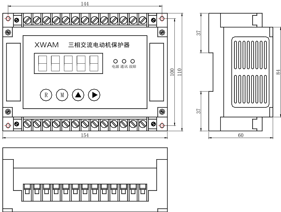
AMDGH-X/E25□ 系列电动机保护器主单元外形及安装孔尺寸
