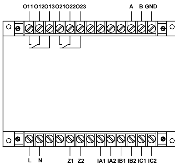
AMDGH-X/E252 系列保护器主单元接线端子图
