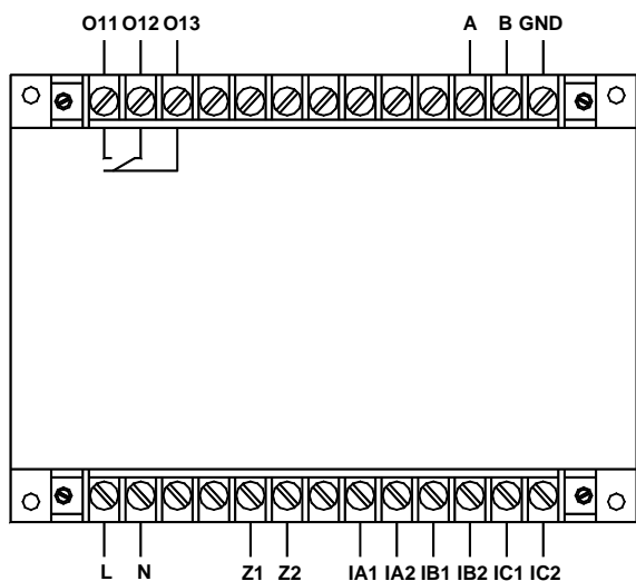
AMDGH-X/E251 系列保护器主单元接线端子图
