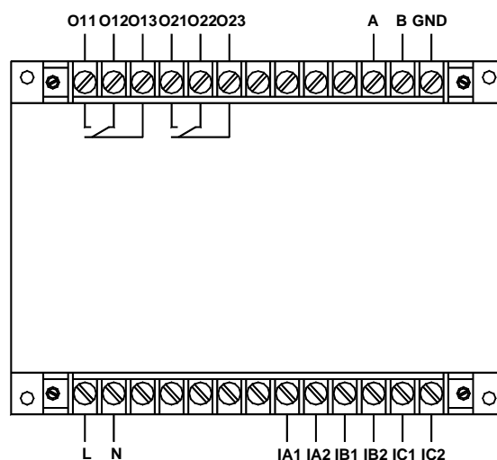
AMDGH-X/E222 系列保护器主单元接线端子图
