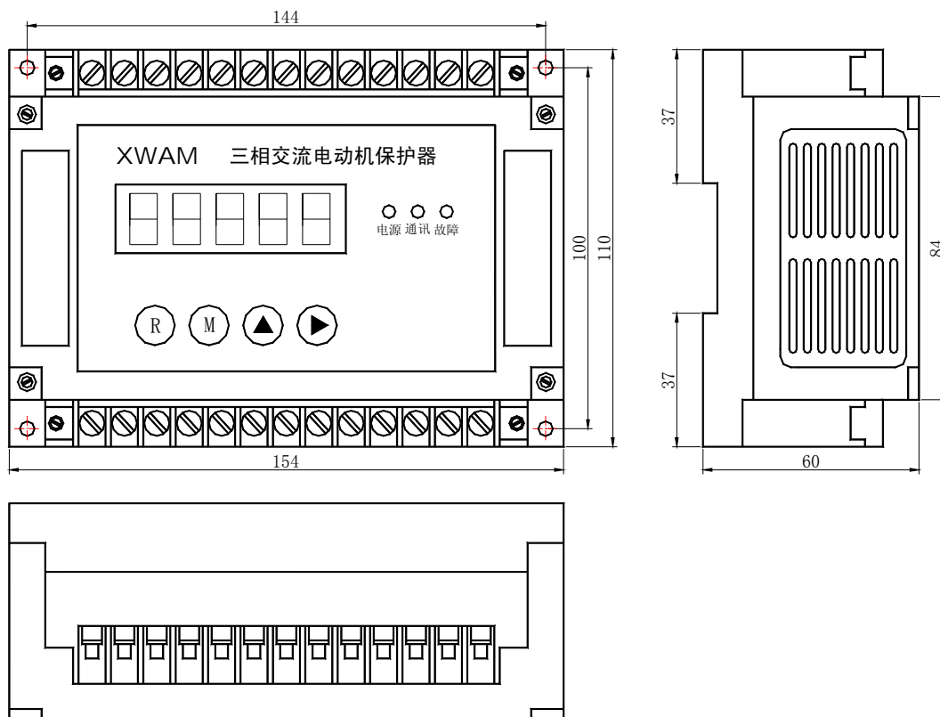
AMDGH-X/E22□ 系列电动机保护器主单元外形及安装孔尺寸
