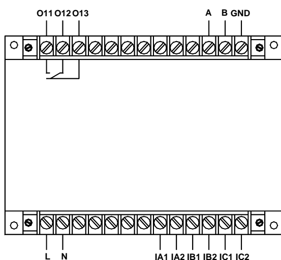
AMDGH-X/E221 系列保护器主单元接线端子图
