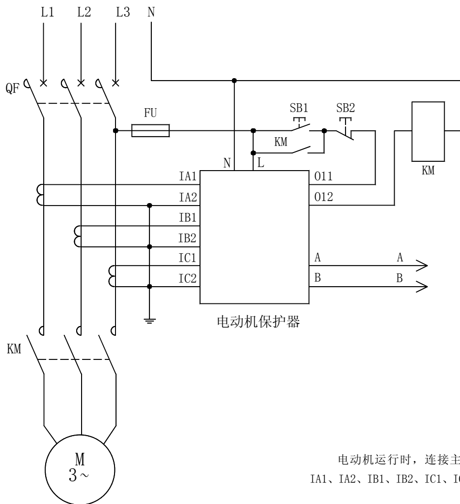
AMDGH-X/E22□ 系列电动机保护器应用电气原理图
