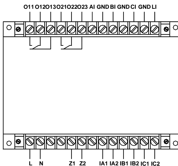
AMDGH-X/E152 系列保护器主单元接线端子图
