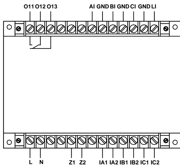
AMDGH-X/E151 系列保护器主单元接线端子图
