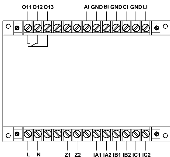
AMDGH-X/E111 系列保护器主单元接线端子图
