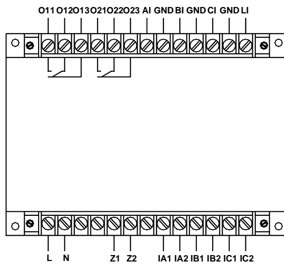
AMDGH-X/E112 系列保护器主单元接线端子图
