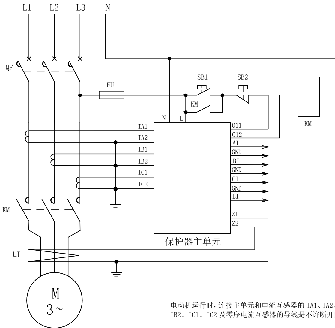
AMDGH-X/E11□ 系列电动机保护器应用电气原理图
