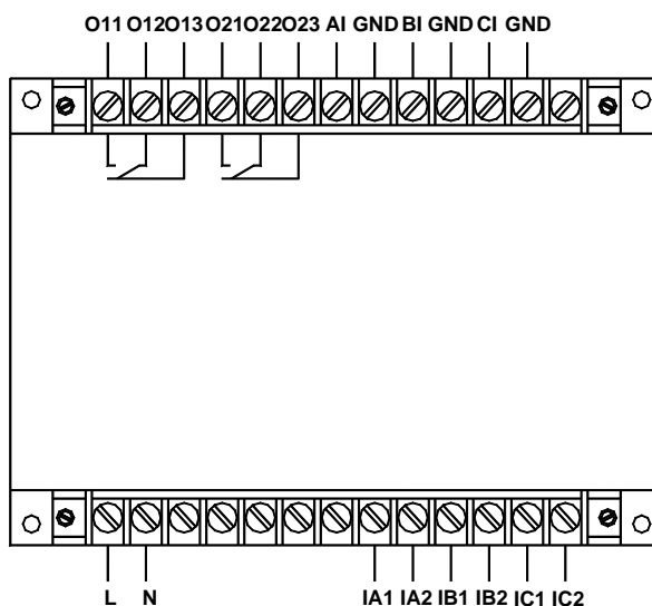
AMDGH-X/E102 系列保护器主单元接线端子图
