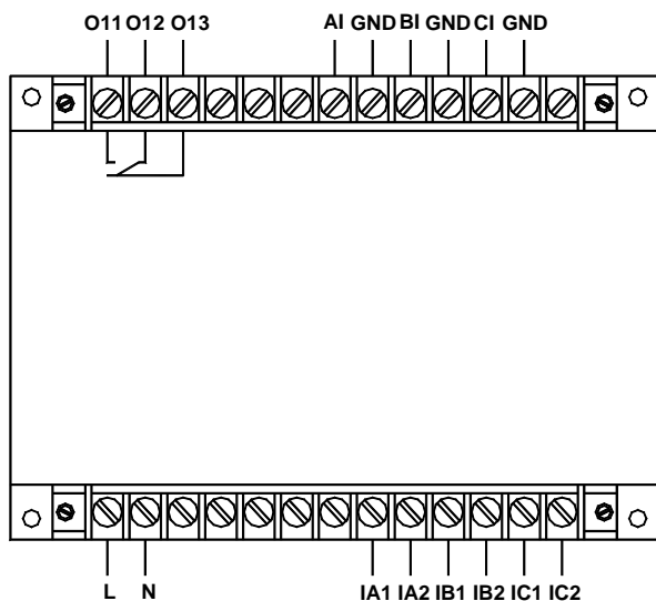
AMDGH-X/E101 系列保护器主单元接线端子图
