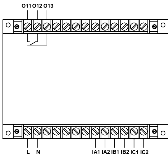
AMDGH-X/E021 系列保护器主单元接线端子图
