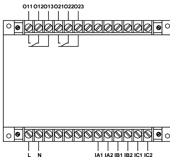
AMDGH-X/E022 系列保护器主单元接线端子图
