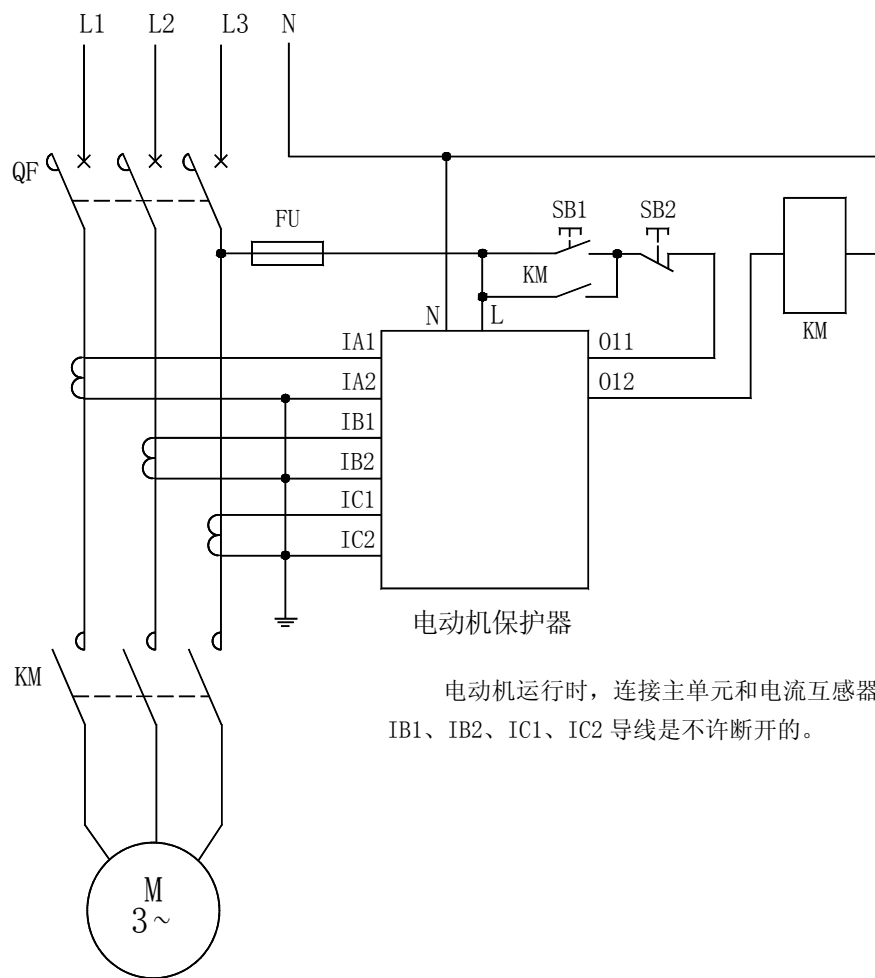
AMDGH-X/E02□ 系列电动机保护器应用电气原理图
