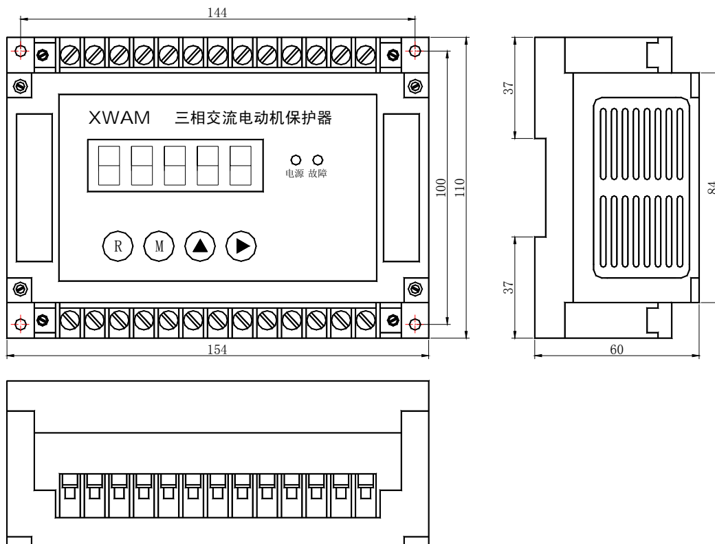
AMDGH-X/E02□ 系列电动机保护器主单元外形及安装孔尺寸
