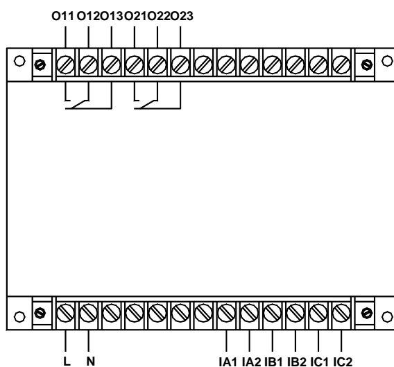
AMDGH-X/E002 系列保护器主单元接线端子图
