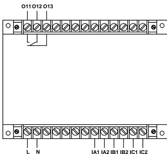
AMDGH-X/E001 系列保护器主单元接线端子图
