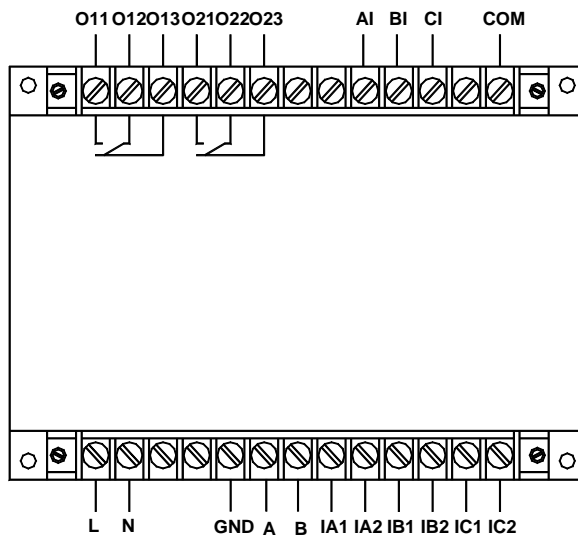
AMDGH-□/C402 系列保护器主单元接线端子图
