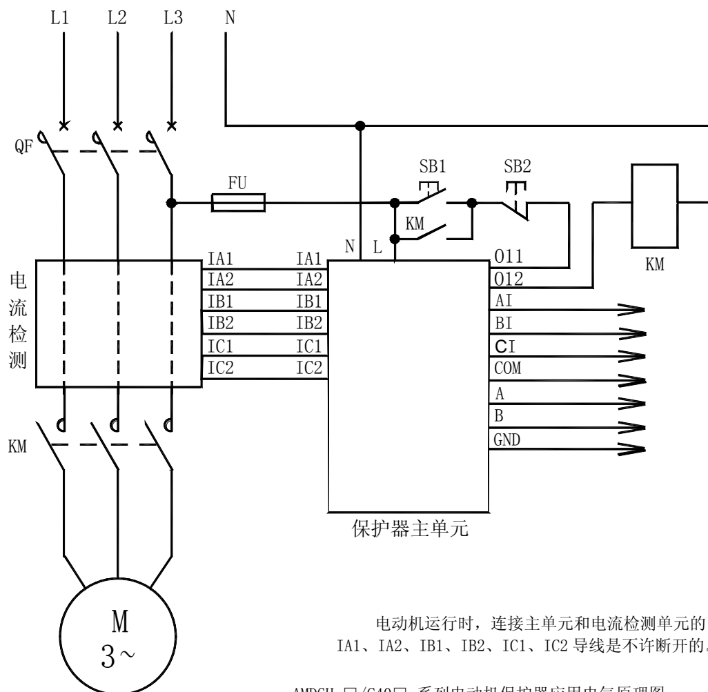
AMDGH-□/□C40□ 系列电动机保护器应用电气原理图
