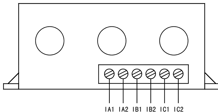
AMDGH-□/C40□ 系列保护器电流检测单元接线端子图
