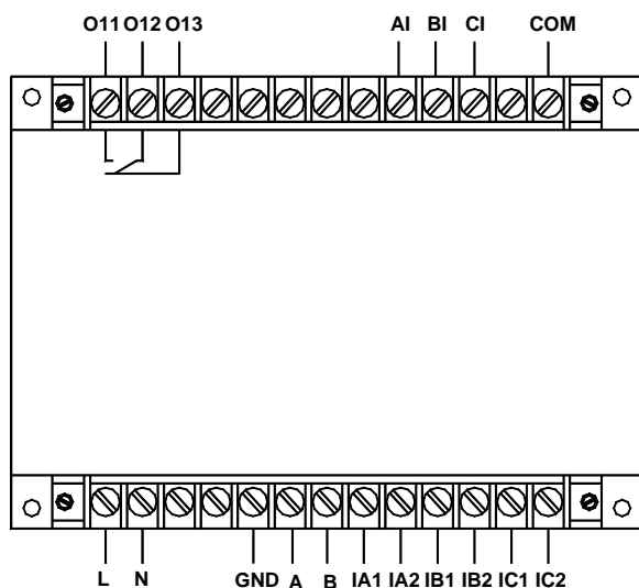
AMDGH-□/C401 系列保护器主单元接线端子图
