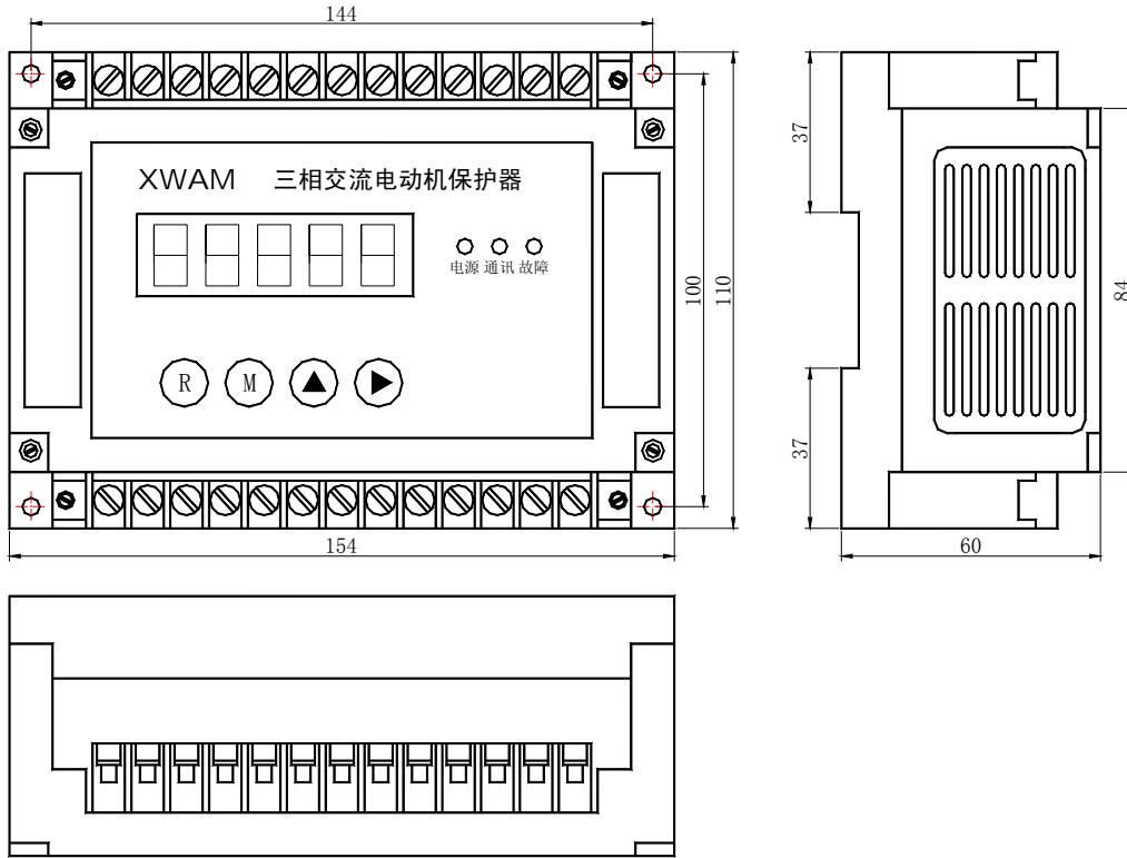
AMDGH-□/□/40□ 系列电动机保护器主单元外形及安装孔尺寸
