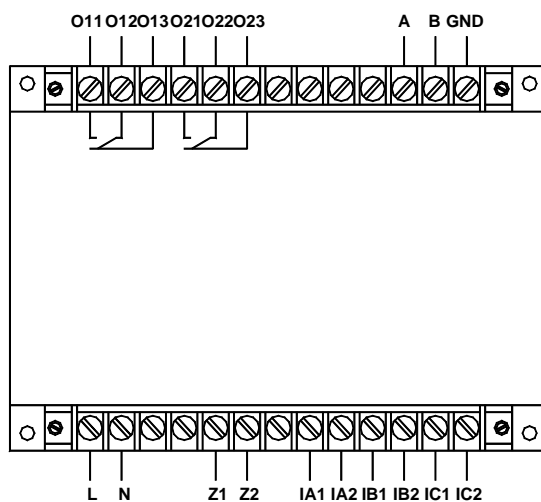
AMDGH-□/ C212 系列保护器主单元接线端子图
