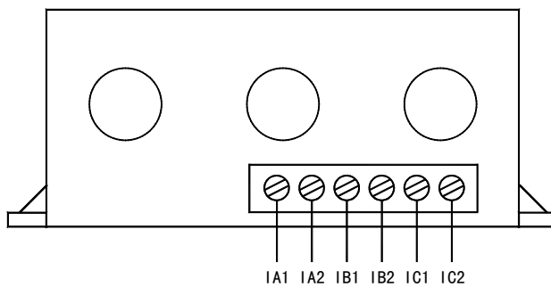
AMDGH-□/ C21□ 系列保护器电流检测单元接线端子图
