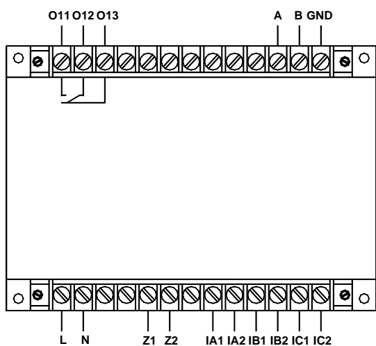
AMDGH-□/ C211 系列保护器主单元接线端子图
