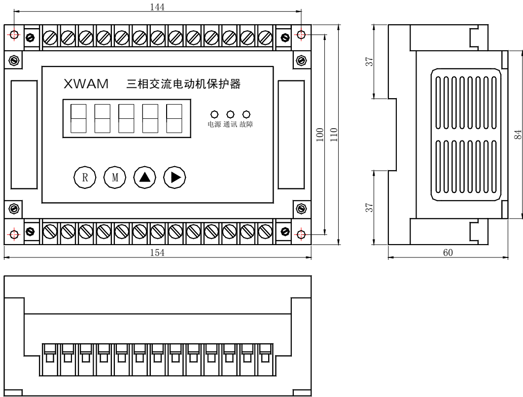
AMDGH-□/□/20□ 系列电动机保护器主单元外形及安装孔尺寸
