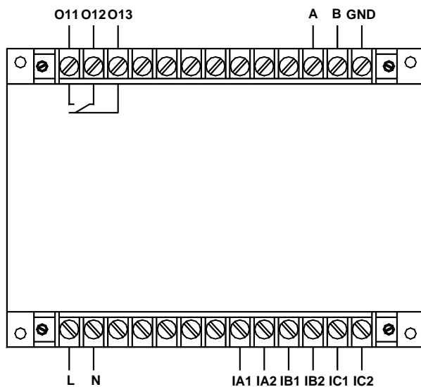
AMDGH-□/201 系列保护器主单元接线端子图
