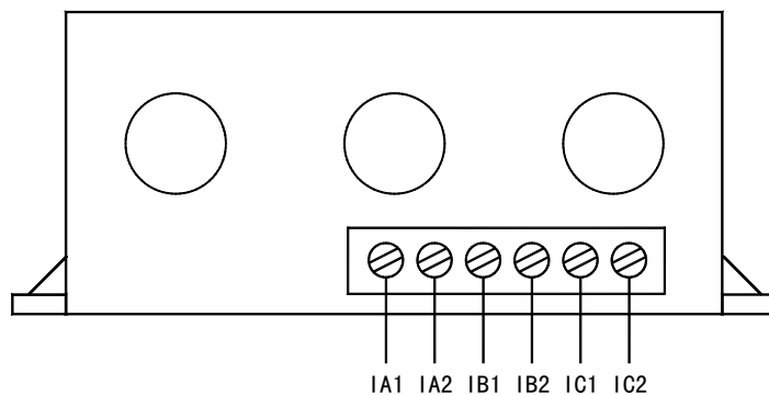
AMDGH-□/20□ 系列保护器电流检测单元接线端子图
