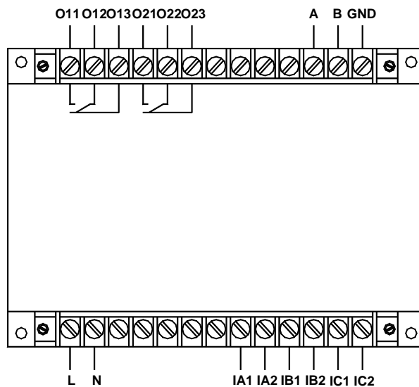
AMDGH-□/202 系列保护器主单元接线端子图
