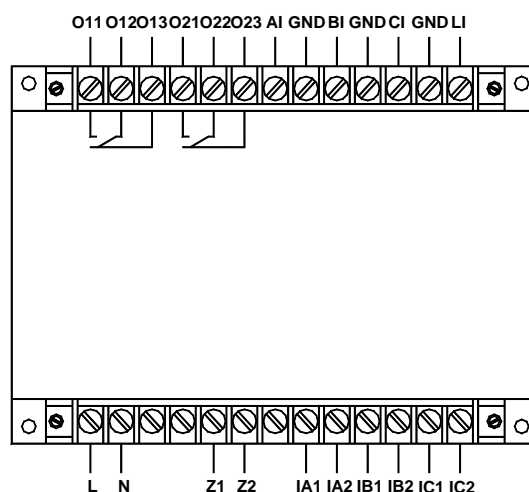
AMDGH-□/□C152 系列保护器主单元接线端子图
