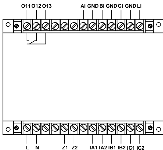
AMDGH-□/□C151 系列保护器主单元接线端子图
