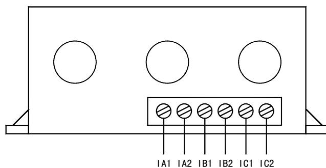
AMDGH-□/ C15□ 系列保护器电流检测单元接线端子图
