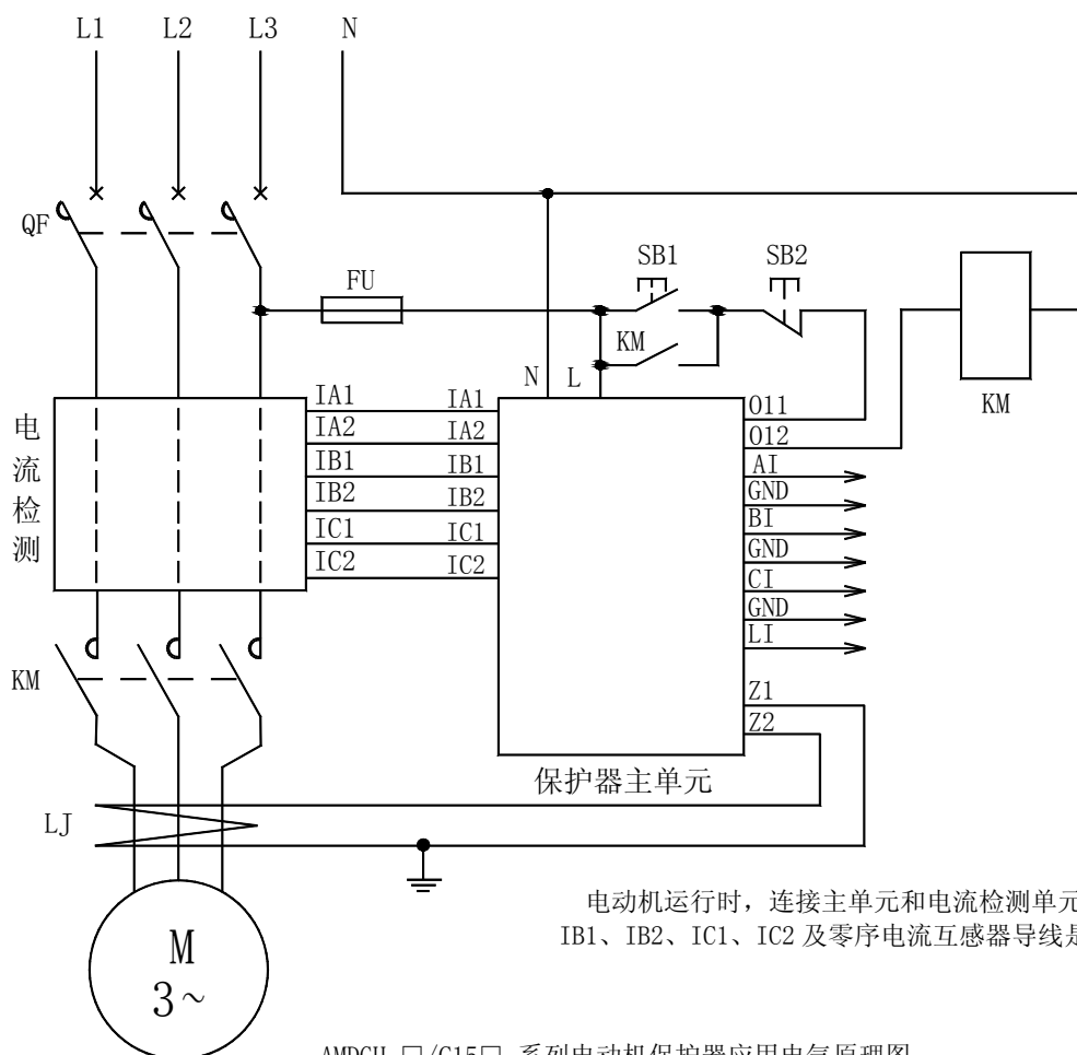
AMDGH-□/ C15□ 系列电动机保护器应用电气原理图
