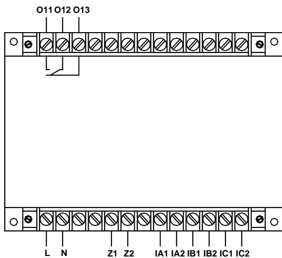
AMDGH-□/CO51 系列保护器主单元接线端子图
