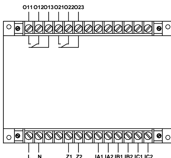
AMDGH-□/CO52 系列保护器主单元接线端子图
