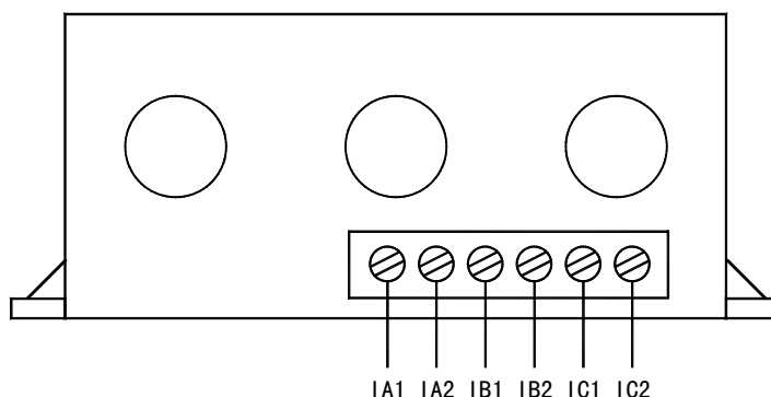
AMDGH-□/CO5□ 系列保护器电流检测单元接线端子图
