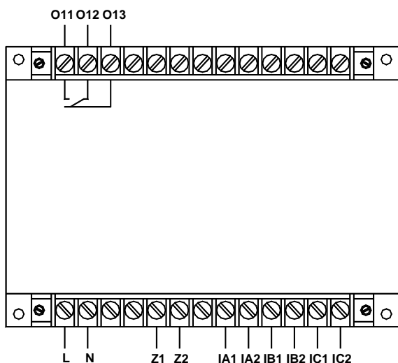
AMDGH-□/CO11 系列保护器主单元接线端子图
