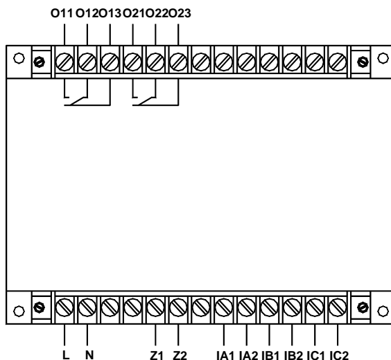
AMDGH-□/CO12 系列保护器主单元接线端子图
