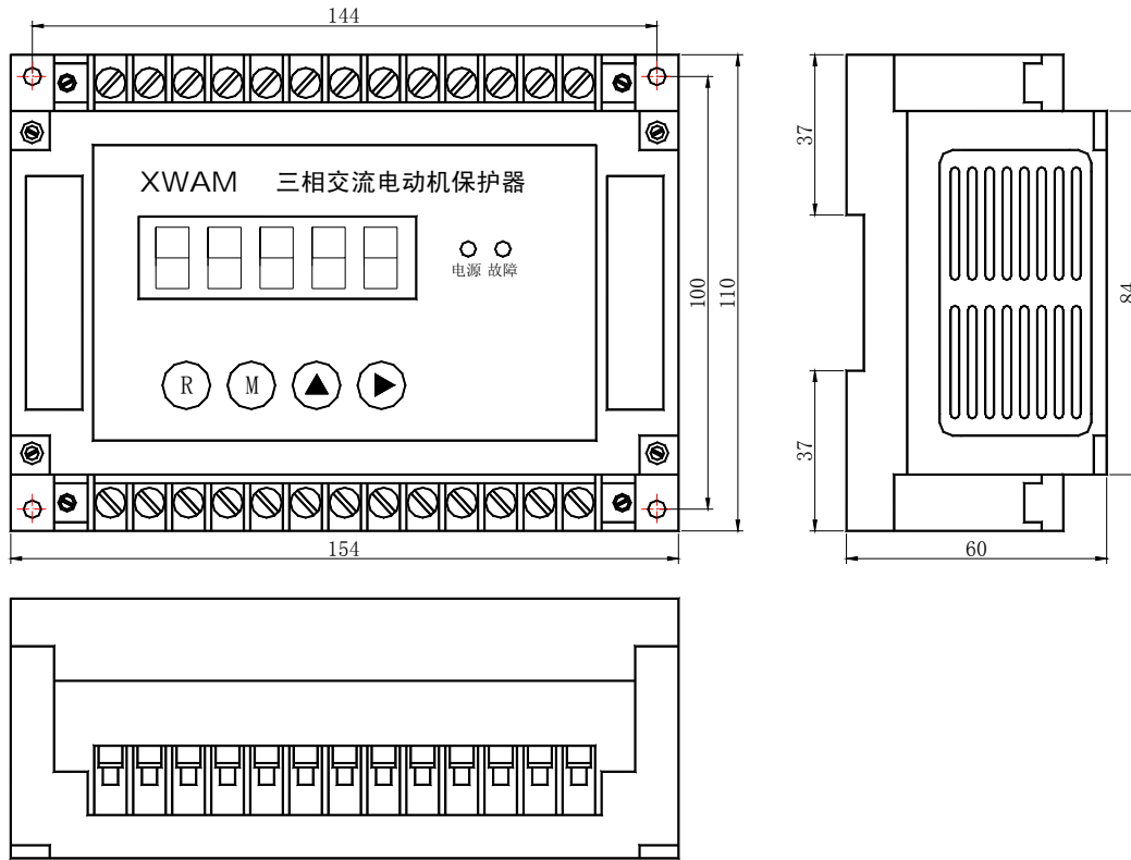
AMDGH-□/CO1□ 系列电动机保护器主单元外形及安装孔尺寸
