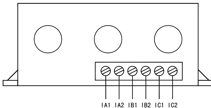
AMDGH-□/CO1□ 系列保护器电流检测单元接线端子图
