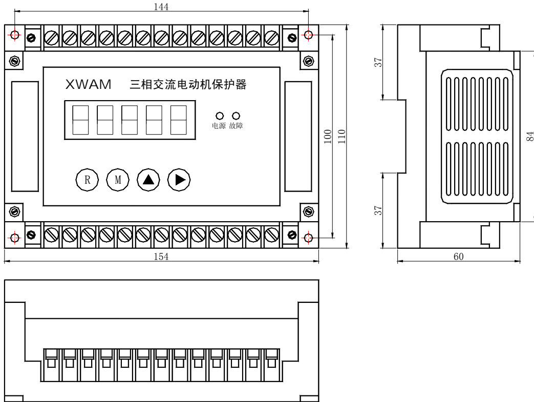
AMDG-X/F821 系列电动机保护器主单元外形及安装孔尺寸
