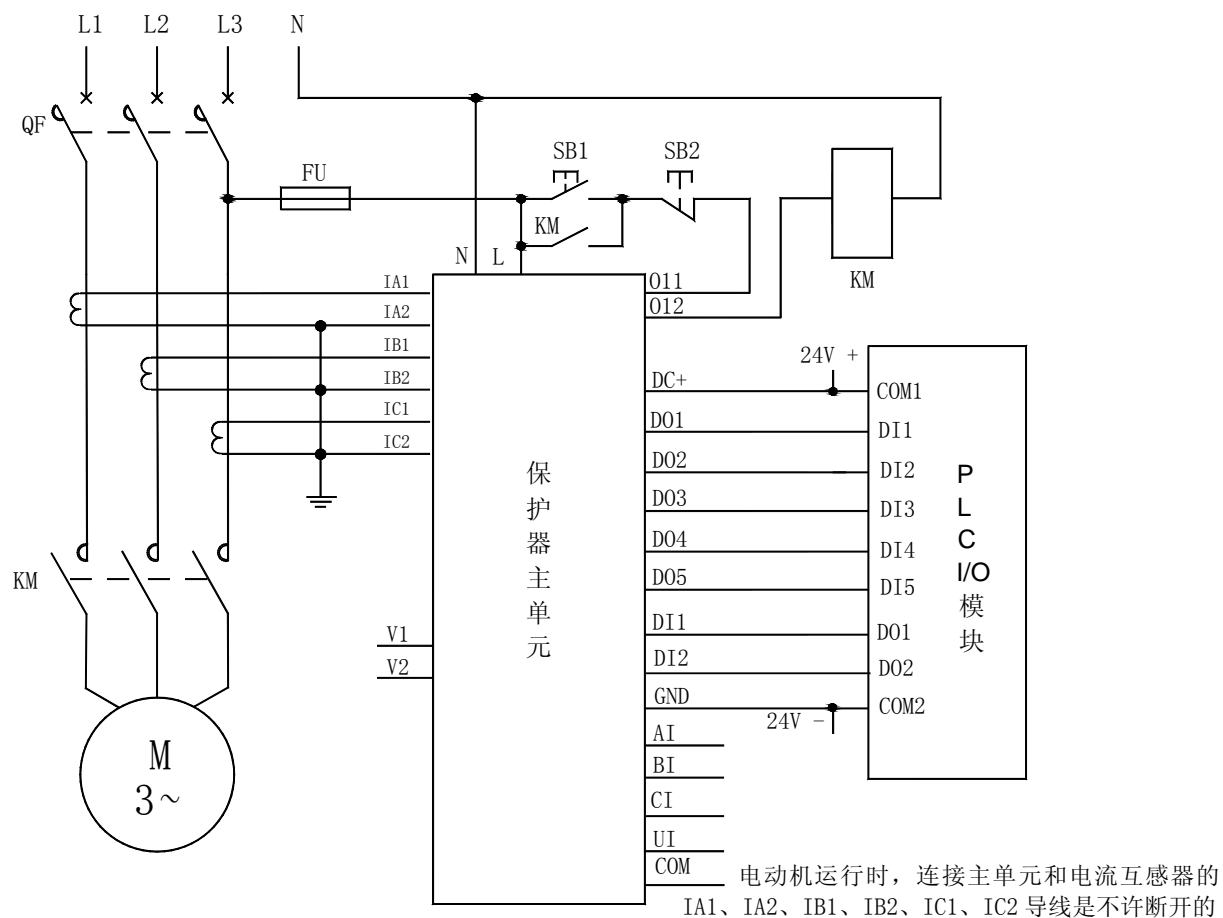
AMDG-X/F821 系列电动机保护器 DO 连接 PLC 电气原理图
