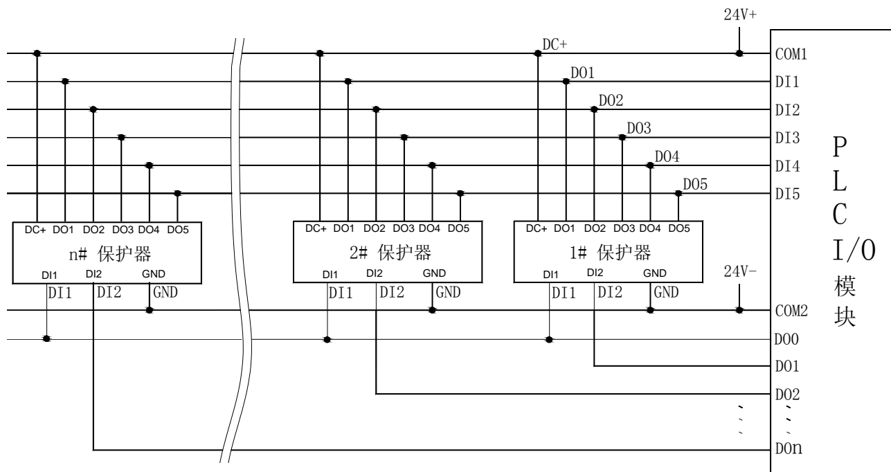
PLC 读取多台 AMDG-X/F821 系列电动机保护器电气原理图
