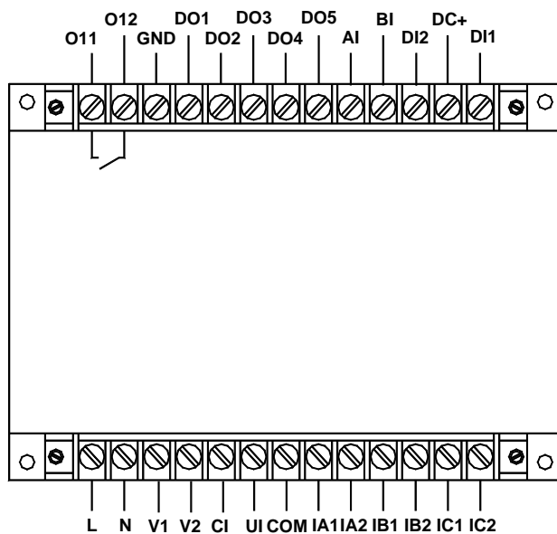
AMDG-X/F821 系列保护器主单元接线端子图
