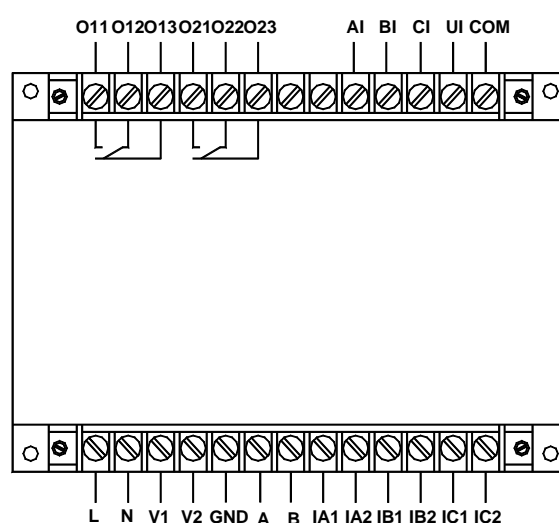
AMDG-X/F442 系列保护器主单元接线端子图
