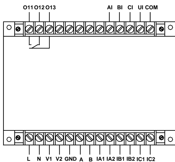
AMDG-X/F441 系列保护器主单元接线端子图
