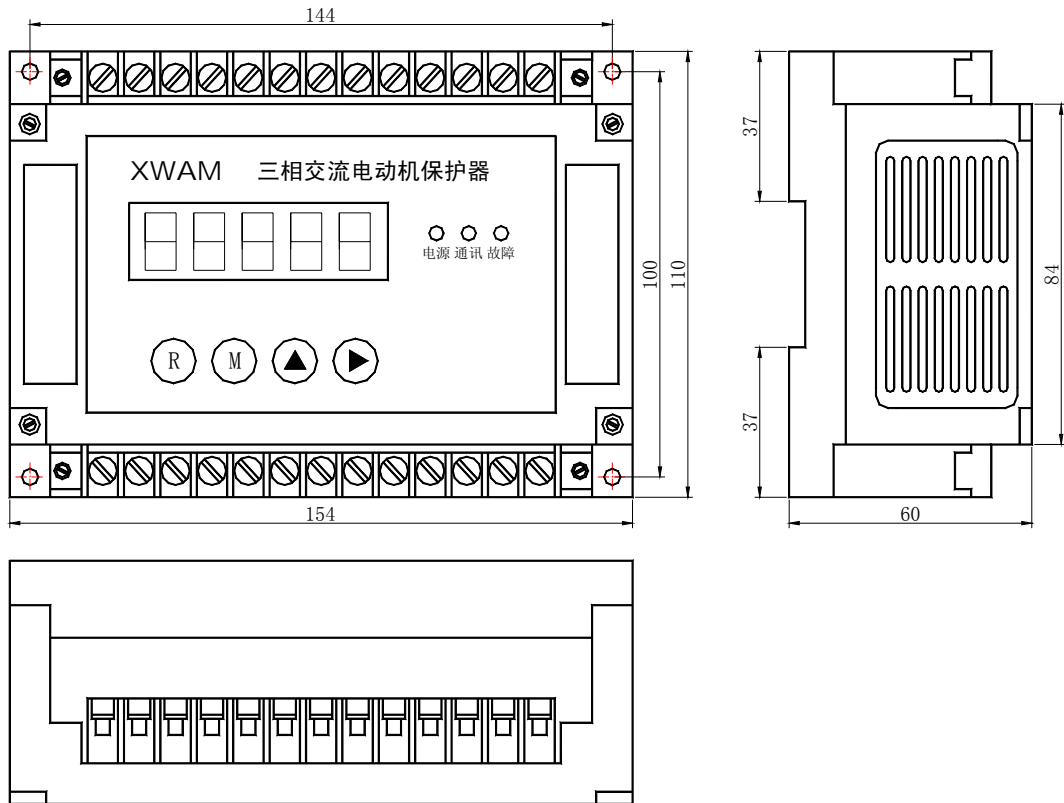
AMDG-X/F44□ 系列电动机保护器主单元外形及安装孔尺寸
