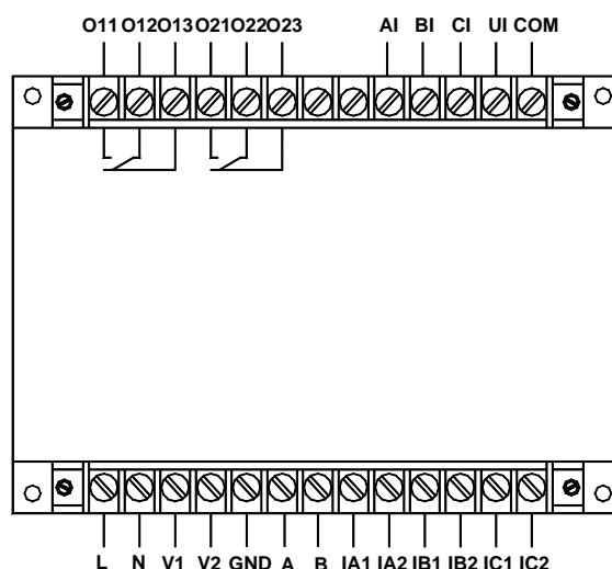
AMDG-X/F432 系列保护器主单元接线端子图
