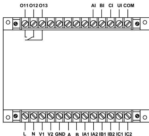
AMDG-X/F431 系列保护器主单元接线端子图
