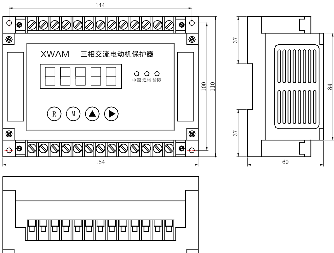
AMDG-X/F43□ 系列电动机保护器主单元外形及安装孔尺寸
