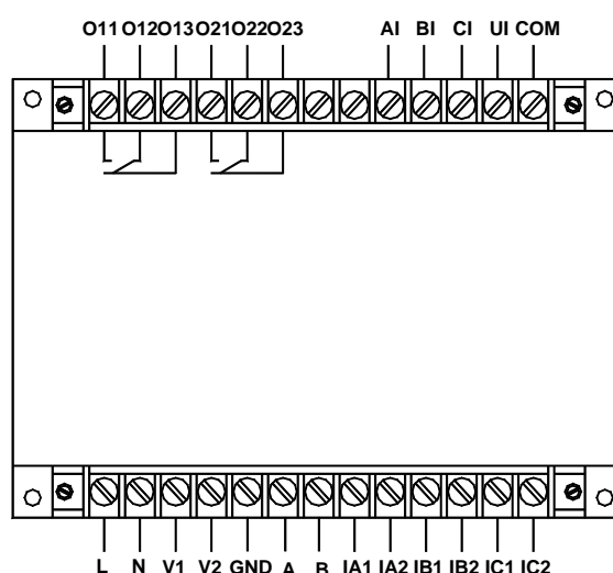
AMDG-X/F402 系列保护器主单元接线端子图
