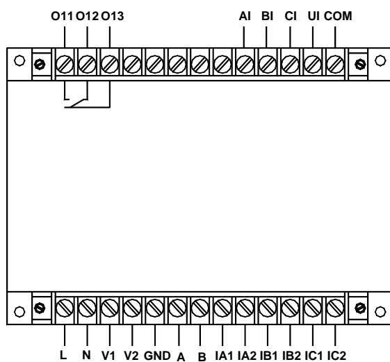
AMDG-X/F401 系列保护器主单元接线端子图
