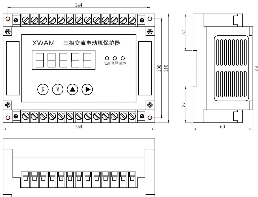
AMDG-X/F40□ 系列电动机保护器主单元外形及安装孔尺寸
