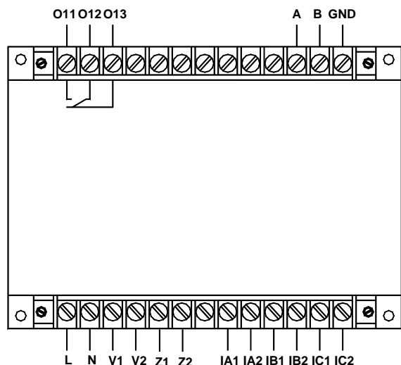
AMDG-X/F361 系列保护器主单元接线端子图
