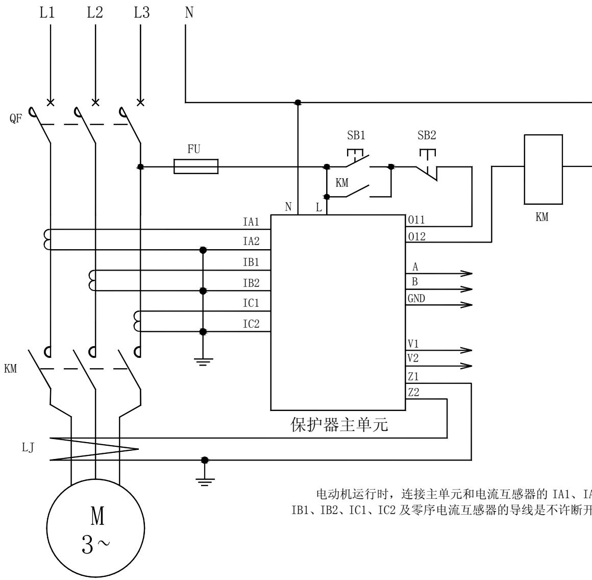
AMDG-X/F36□ 系列电动机保护器应用电气原理图
