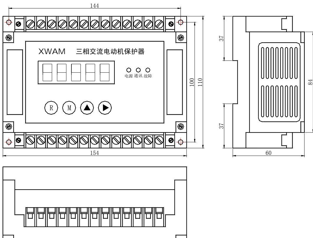
AMDG-X/F36□ 系列电动机保护器主单元外形及安装孔尺寸
