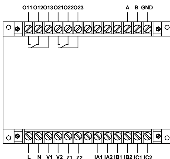
AMDG-X/F362 系列保护器主单元接线端子图
