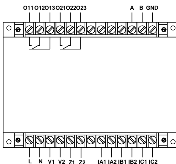
AMDG-X/F352 系列保护器主单元接线端子图
