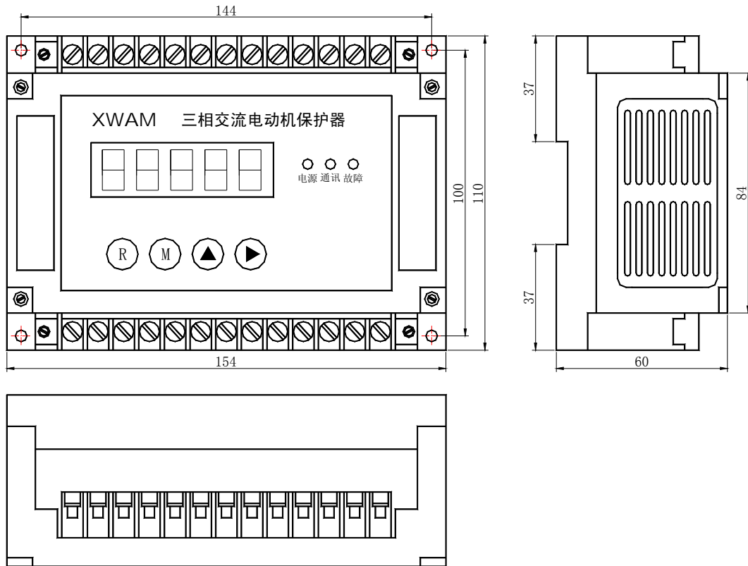
AMDG-X/F35□ 系列电动机保护器主单元外形及安装孔尺寸
