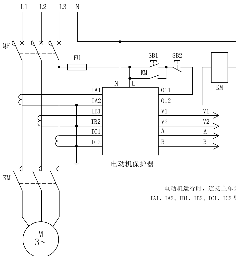
AMDG-X/F34□ 系列电动机保护器应用电气原理图
