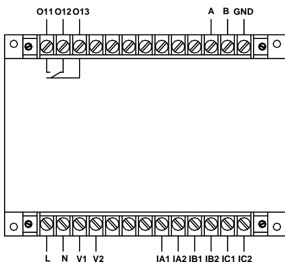
AMDG-X/F341 系列保护器主单元接线端子图
