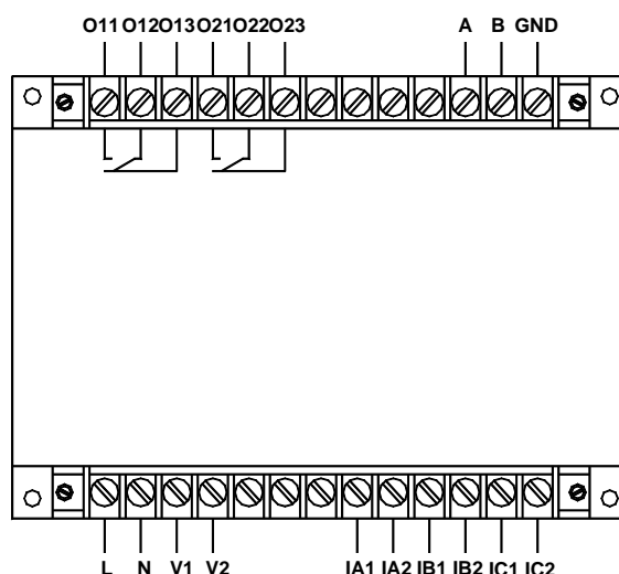
AMDG-X/F342 系列保护器主单元接线端子图
