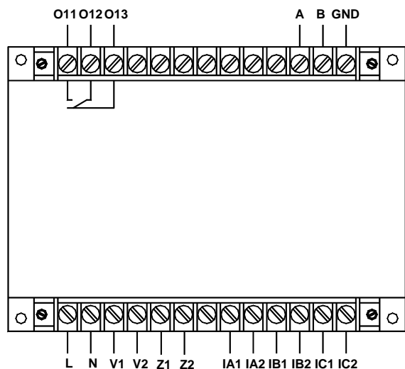
AMDG-X/F311 系列保护器主单元接线端子图
