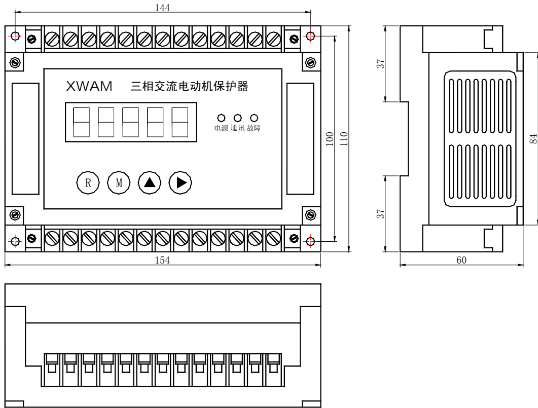
AMDG-X/F31□ 系列电动机保护器主单元外形及安装孔尺寸
