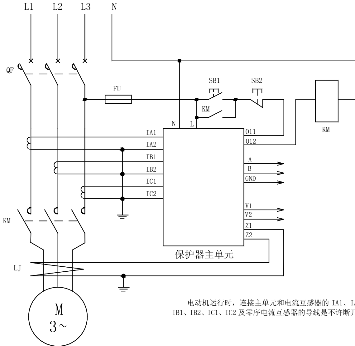
AMDG-X/F31□ 系列电动机保护器应用电气原理图
