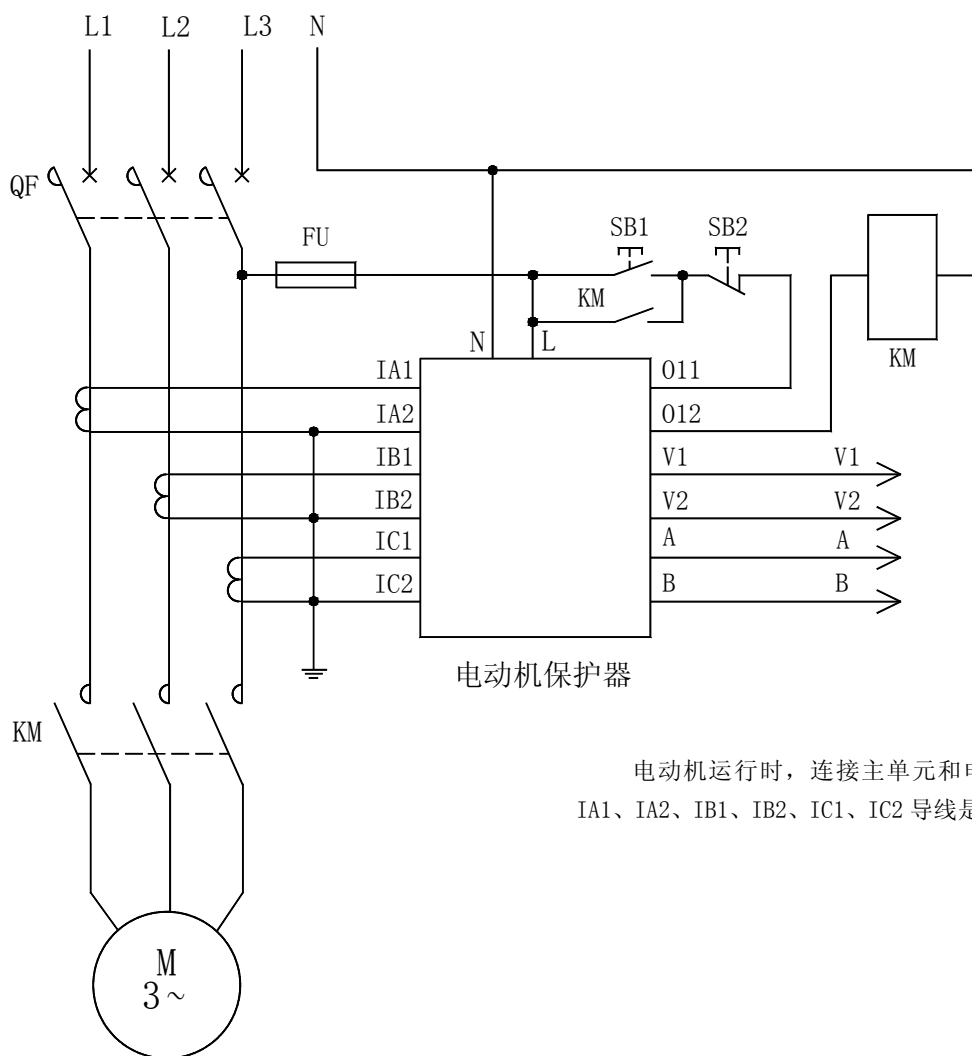
AMDG-X/F30□ 系列电动机保护器应用电气原理图
