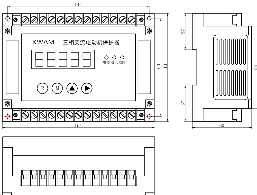
AMDG-X/F30□ 系列电动机保护器主单元外形及安装孔尺寸
