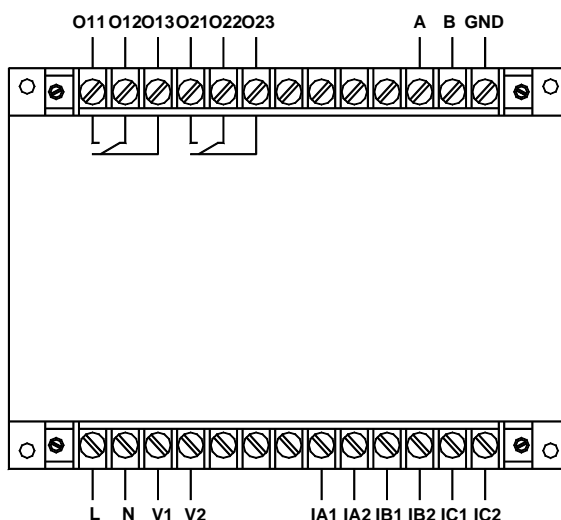
AMDG-X/F302 系列保护器主单元接线端子图
