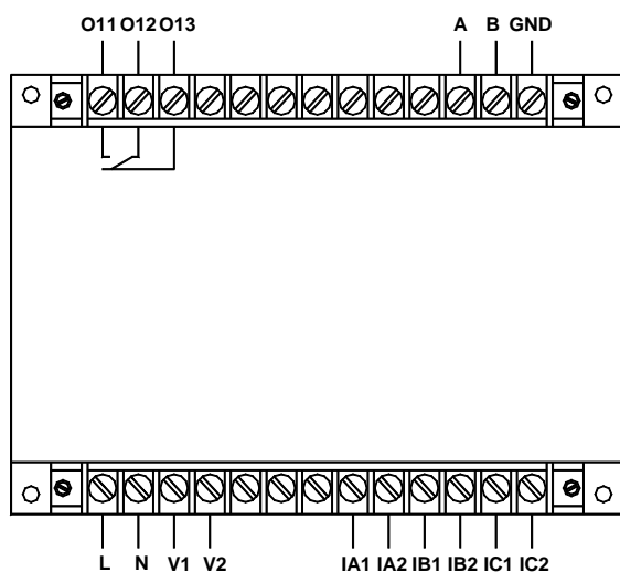
AMDG-X/F301 系列保护器主单元接线端子图
