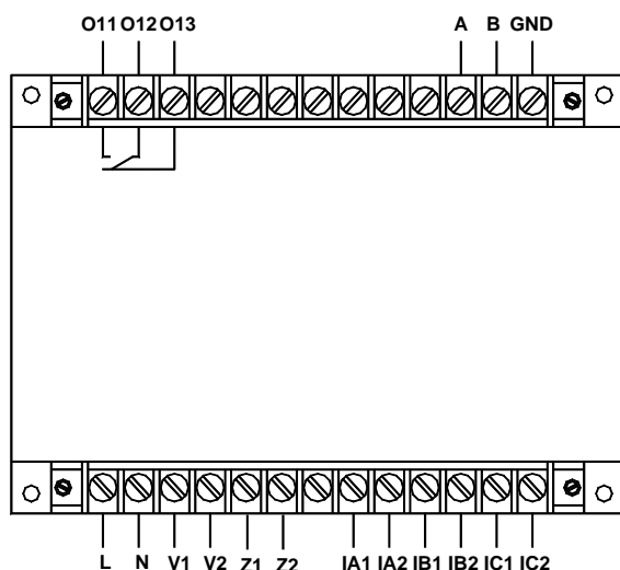
AMDG-X/F261 系列保护器主单元接线端子图
