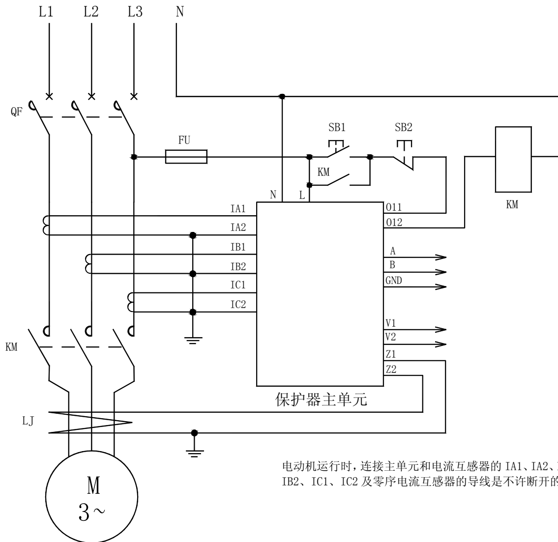
AMDG-X/F26□ 系列电动机保护器应用电气原理图
