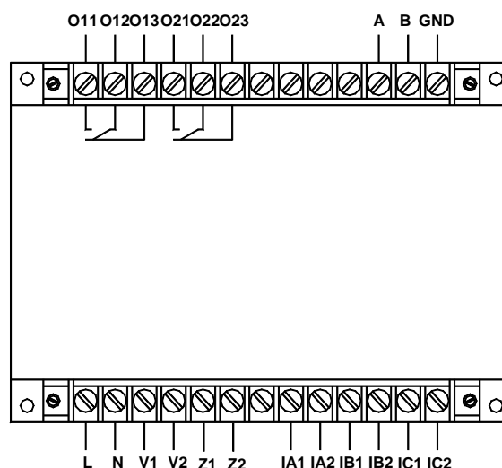
AMDG-X/F262 系列保护器主单元接线端子图
