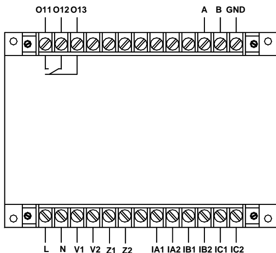
AMDG-X/F251 系列保护器主单元接线端子图
