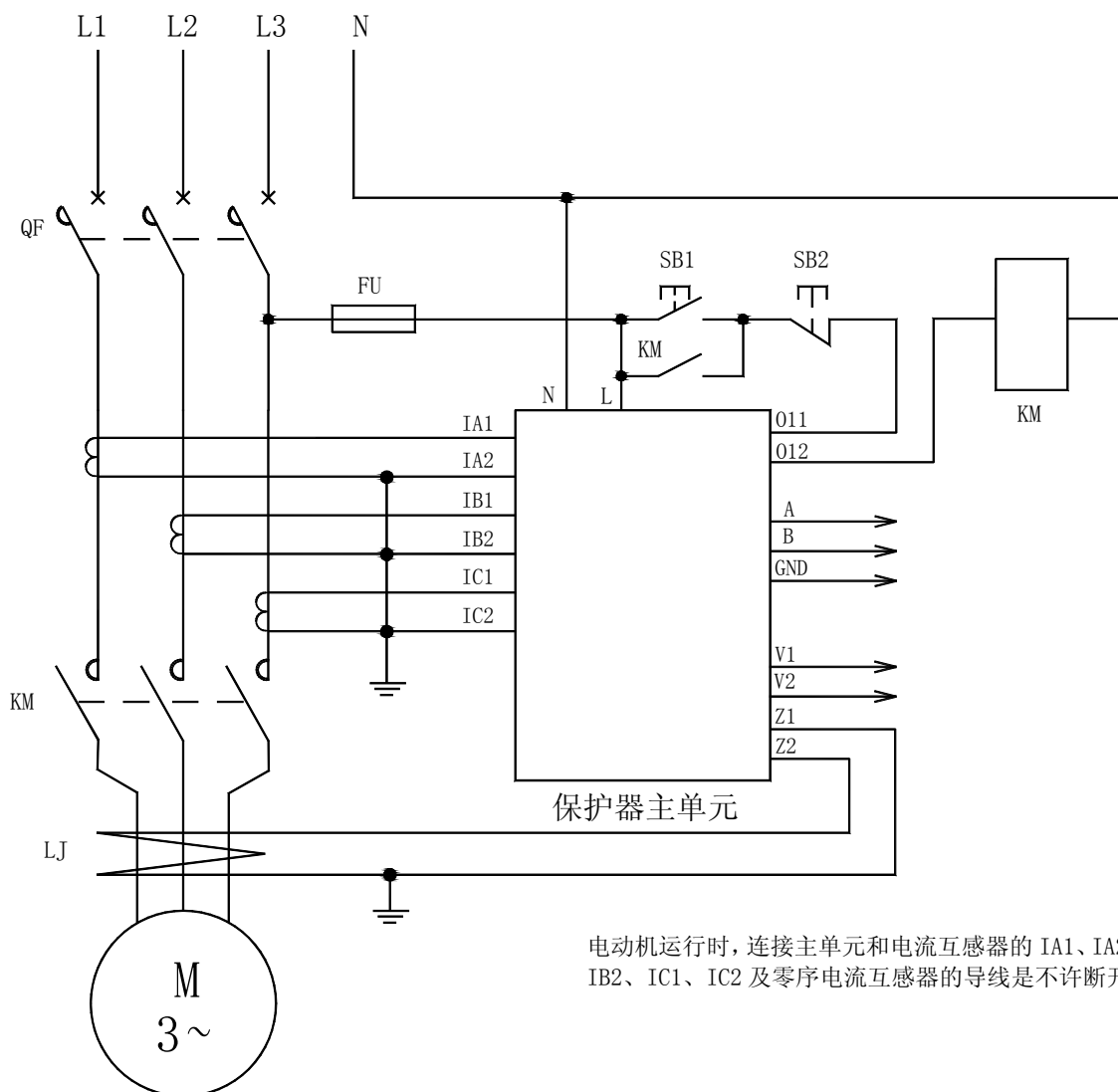
AMDG-X/F25□ 系列电动机保护器应用电气原理图
