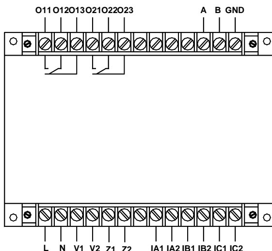
AMDG-X/F252 系列保护器主单元接线端子图
