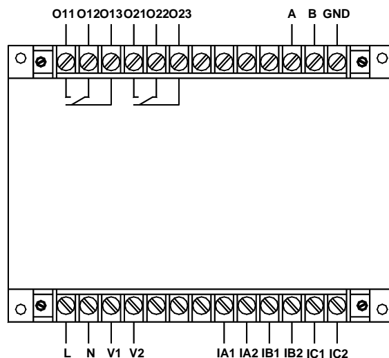
AMDG-X/F242 系列保护器主单元接线端子图
