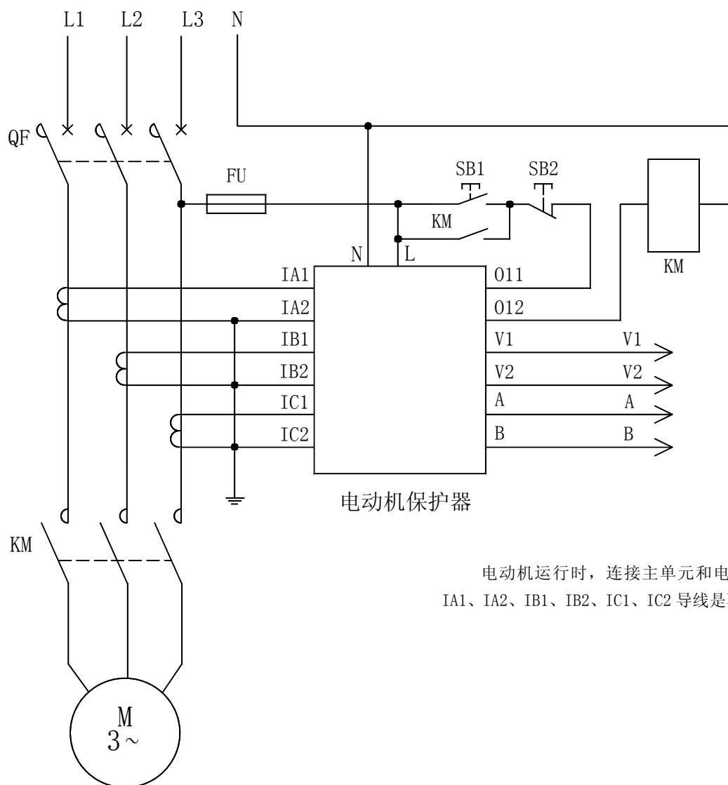
AMDG-X/F24□ 系列电动机保护器应用电气原理图
