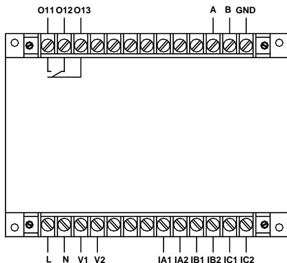
AMDG-X/F241 系列保护器主单元接线端子图
