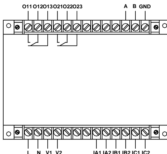
AMDG-X/F232 系列保护器主单元接线端子图
