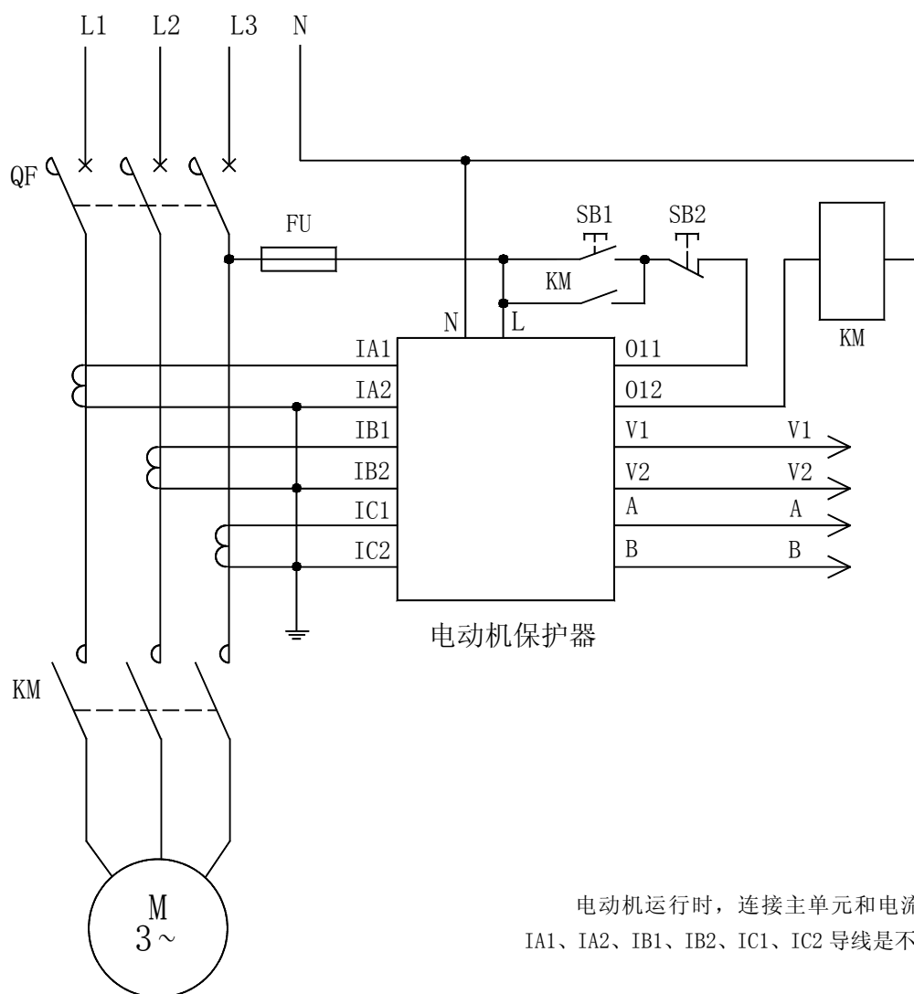
AMDG-X/F23□ 系列电动机保护器应用电气原理图
