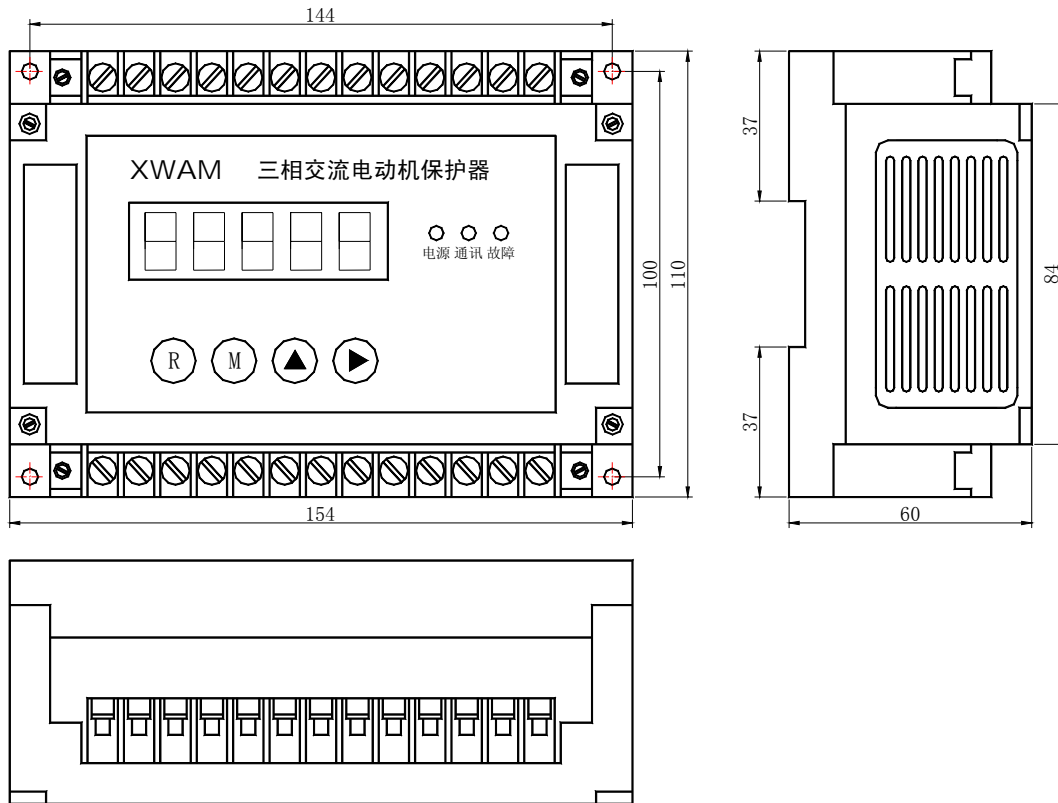
AMDG-X/F23□ 系列电动机保护器主单元外形及安装孔尺寸
