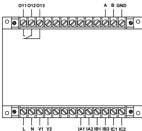
AMDG-X/F231 系列保护器主单元接线端子图
