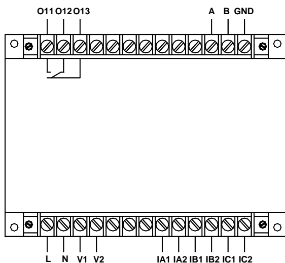
AMDG-X/F221 系列保护器主单元接线端子图
