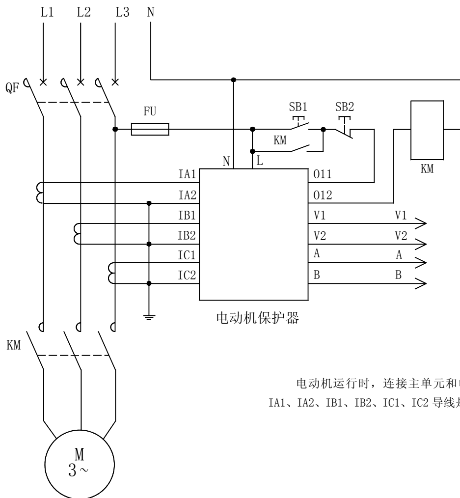
AMDG-X/F22□ 系列电动机保护器应用电气原理图
