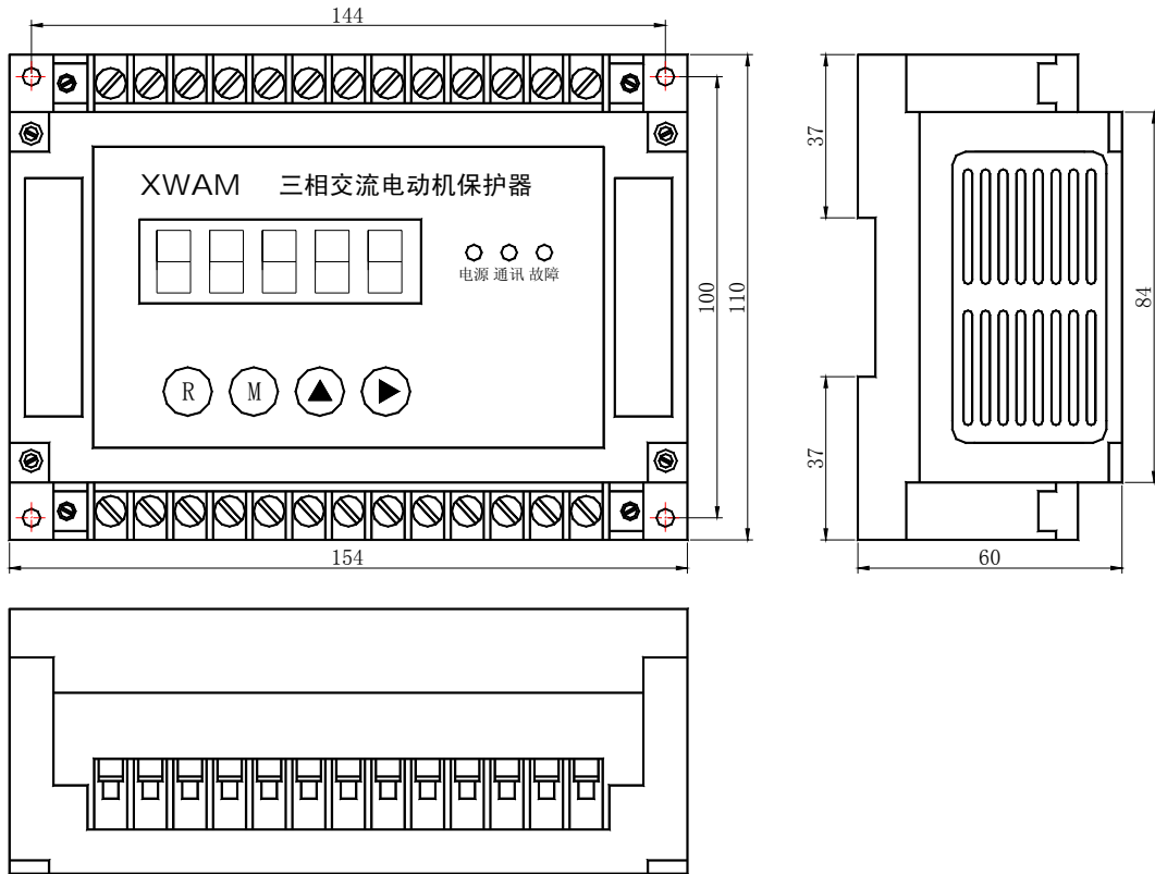
AMDG-X/F22□ 系列电动机保护器主单元外形及安装孔尺寸
