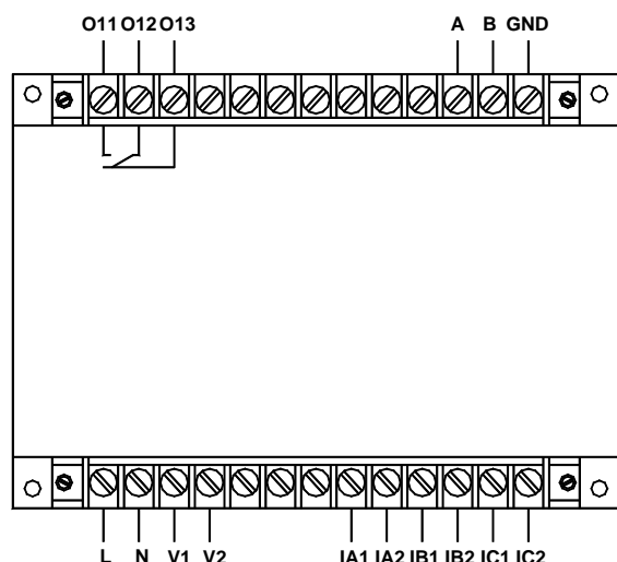
AMDG-X/F201 系列保护器主单元接线端子图
