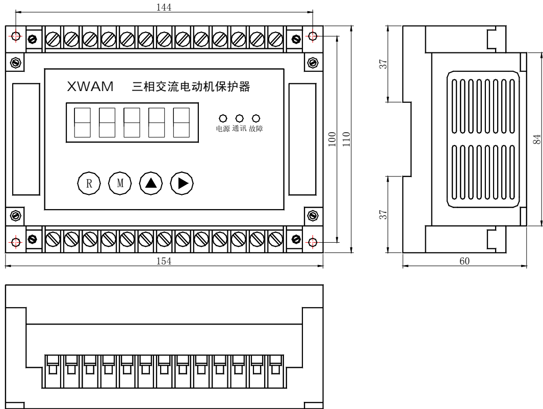
AMDG-X/F20□ 系列电动机保护器主单元外形及安装孔尺寸
