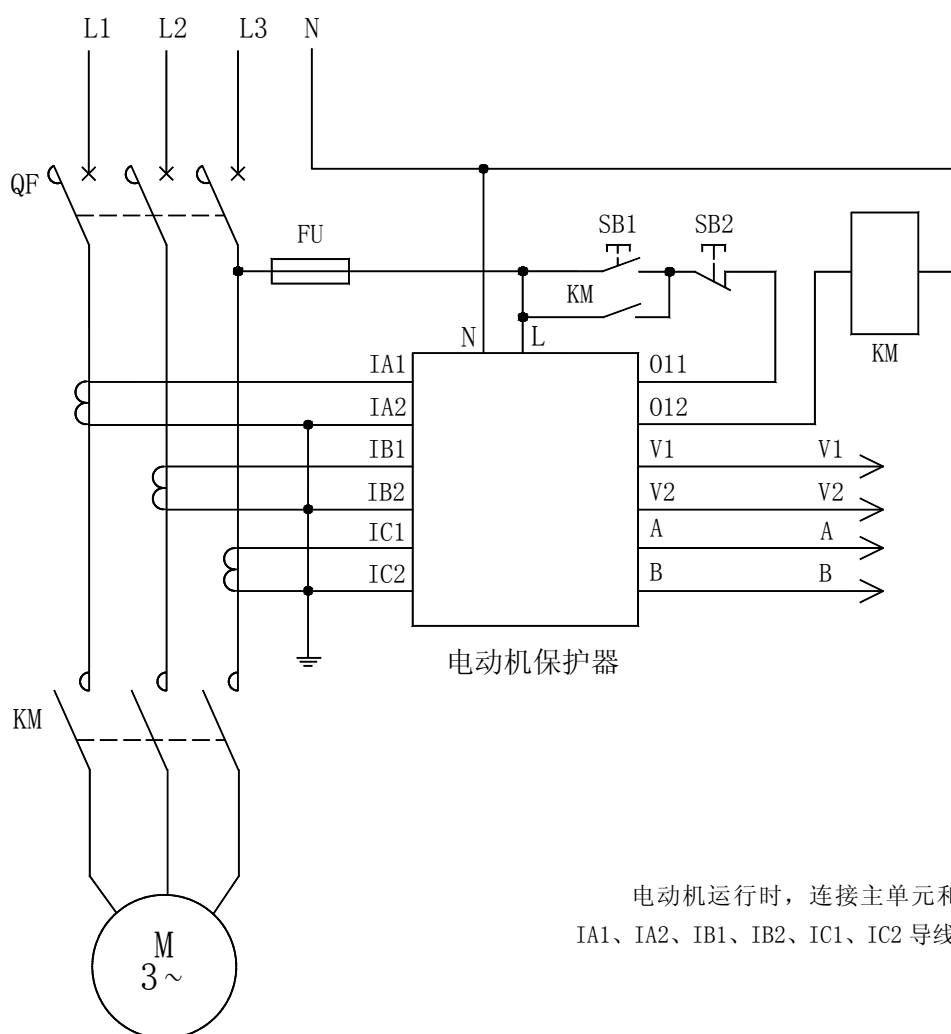
AMDG-X/F20□ 系列电动机保护器应用电气原理图
