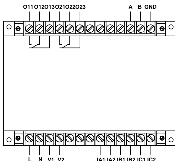
AMDG-X/F202 系列保护器主单元接线端子图
