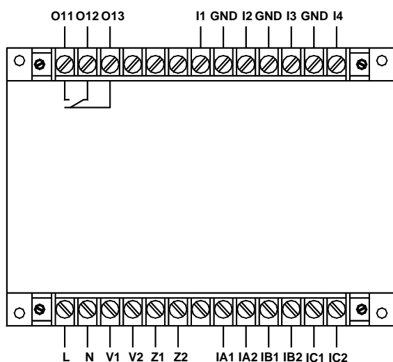
AMDG-X/F171 系列保护器主单元接线端子图
