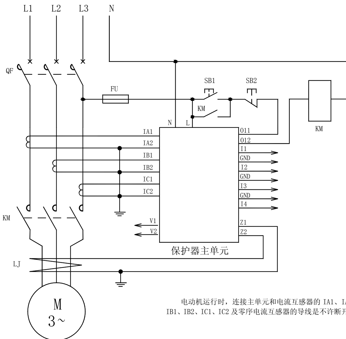
AMDG-X/F17□ 系列电动机保护器应用电气原理图
