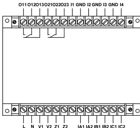
AMDG-X/F172 系列保护器主单元接线端子图
