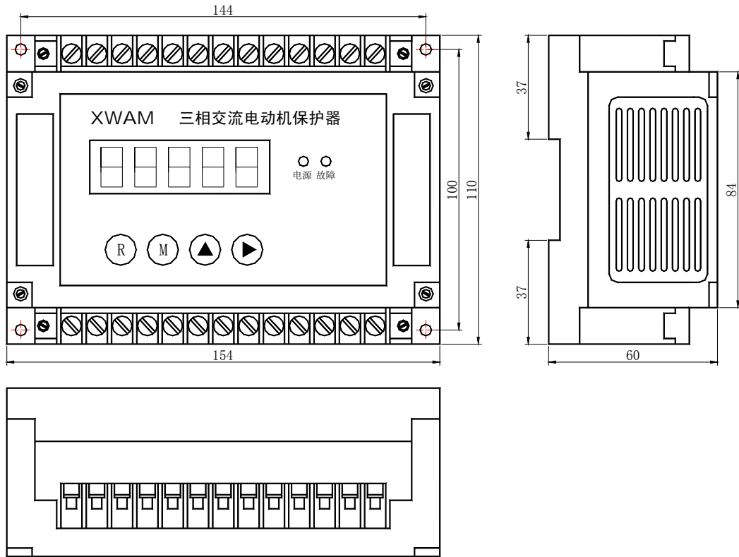
AMDG-X/F17□ 系列电动机保护器主单元外形及安装孔尺寸
