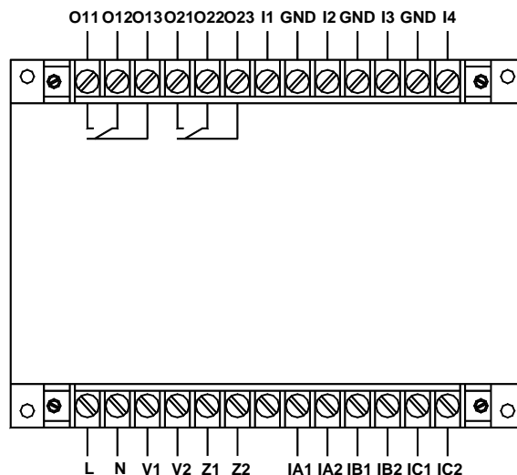
AMDG-X/F162 系列保护器主单元接线端子图
