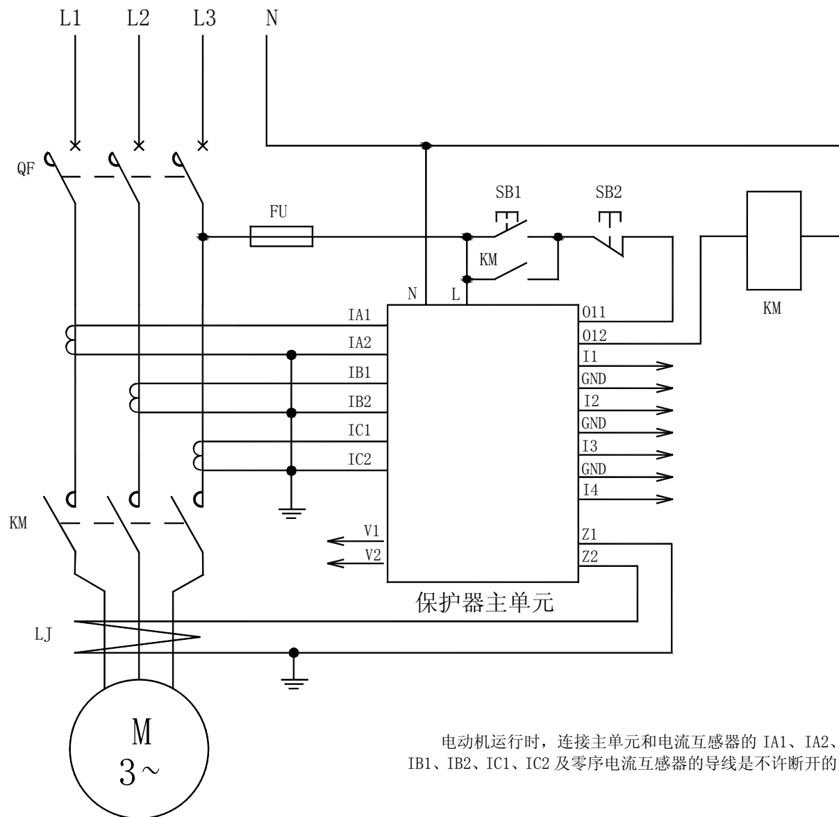
AMDG-X/F16□ 系列电动机保护器应用电气原理图
