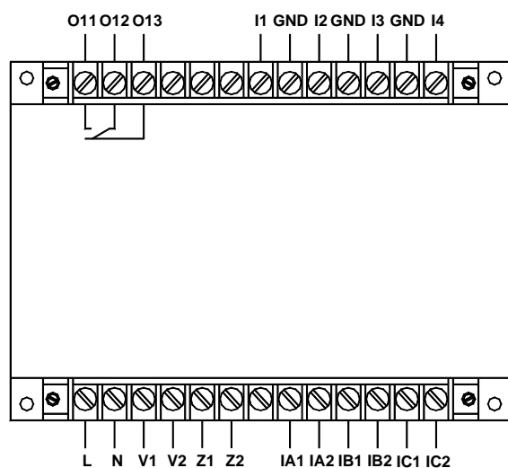
AMDG-X/F161 系列保护器主单元接线端子图
