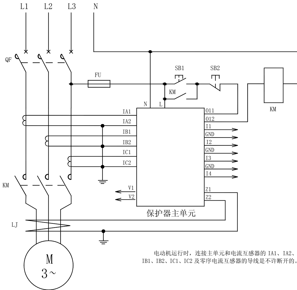
AMDG-X/F15□ 系列电动机保护器应用电气原理图
