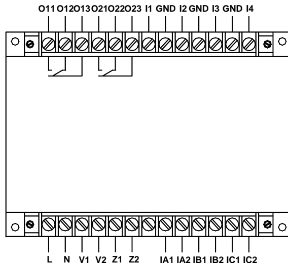
AMDG-X/F152 系列保护器主单元接线端子图
