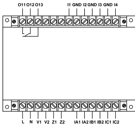
AMDG-X/F151 系列保护器主单元接线端子图
