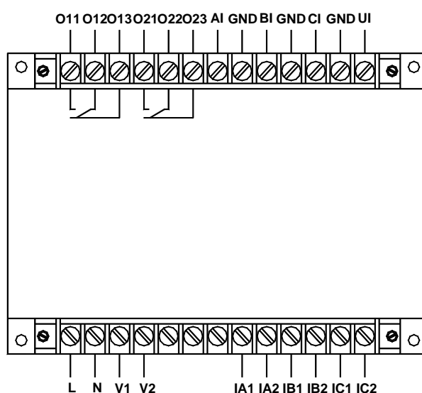
AMDG-X/F142 系列保护器主单元接线端子图
