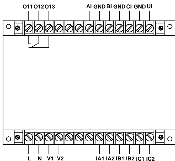
AMDG-X/F141 系列保护器主单元接线端子图 沈阳新维自动化有限公司
