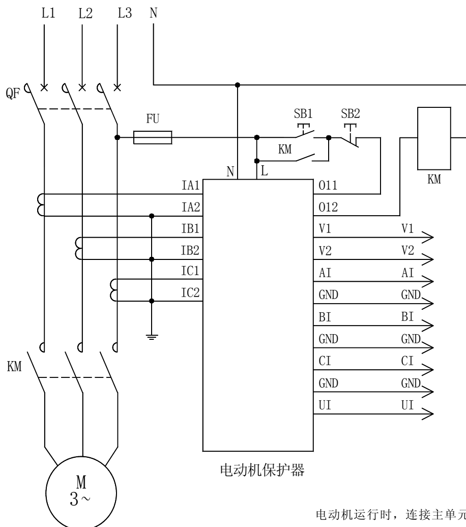
AMDG-X/F13□ 系列电动机保护器应用电气原理图
