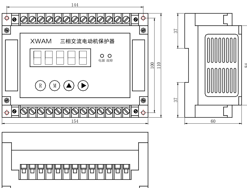
AMDG-X/F13□ 系列电动机保护器主单元外形及安装孔尺寸
