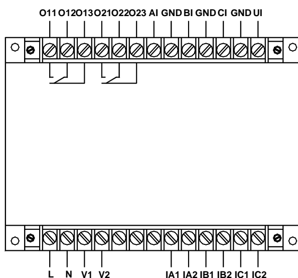
AMDG-X/F132 系列保护器主单元接线端子图
