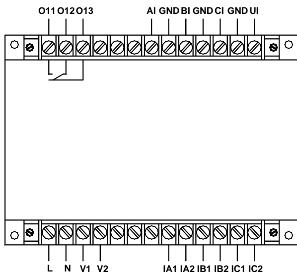
AMDG-X/F131 系列保护器主单元接线端子图
