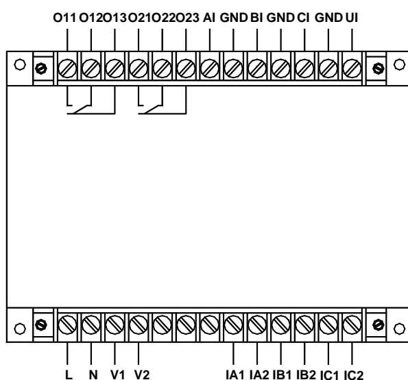
AMDG-X/F122 系列保护器主单元接线端子图
