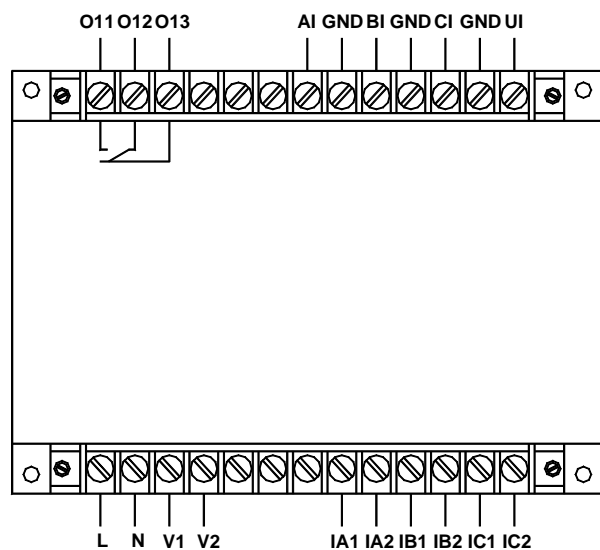
AMDG-X/F121 系列保护器主单元接线端子图
