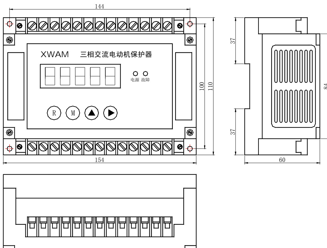
AMDG-X/F12□ 系列电动机保护器主单元外形及安装孔尺寸
