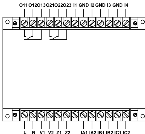
AMDG-X/F112 系列保护器主单元接线端子图
