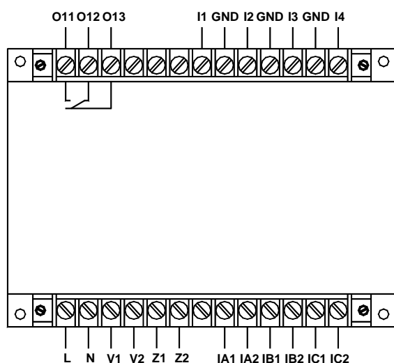
AMDG-X/F111 系列保护器主单元接线端子图
