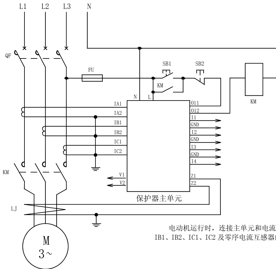
AMDG-X/F11□ 系列电动机保护器应用电气原理图
