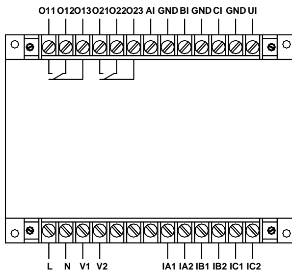
AMDG-X/F102 系列保护器主单元接线端子图 HTTP://WWW.SY-XINWEI.COM
