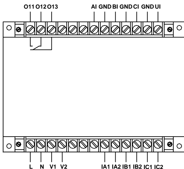
AMDG-X/F101 系列保护器主单元接线端子图 沈阳新维自动化有限公司
