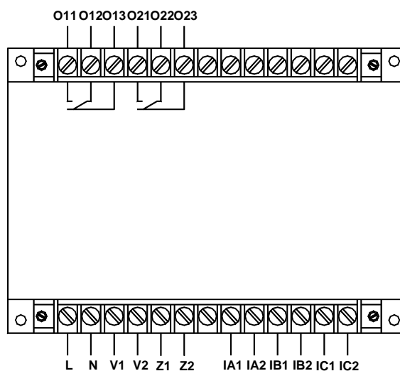
AMDG-X/F072 系列保护器主单元接线端子图
