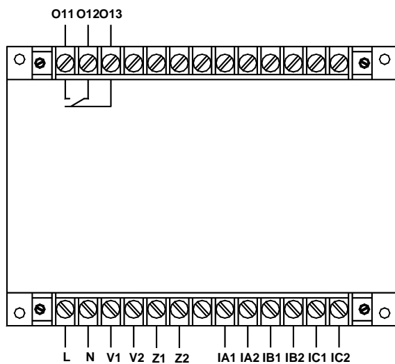
AMDG-X/F071 系列保护器主单元接线端子图
