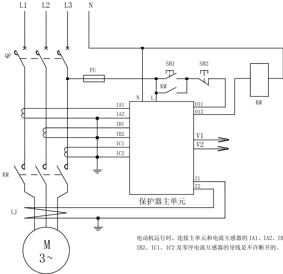
AMDG-X/F07□ 系列电动机保护器应用电气原理图
