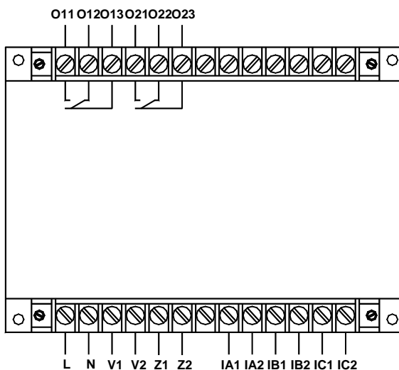
AMDG-X/F062 系列保护器主单元接线端子图
