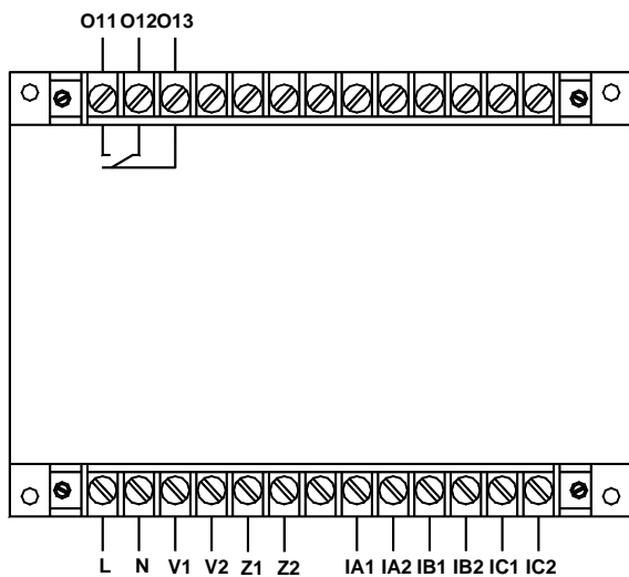
AMDG-X/F061 系列保护器主单元接线端子图
