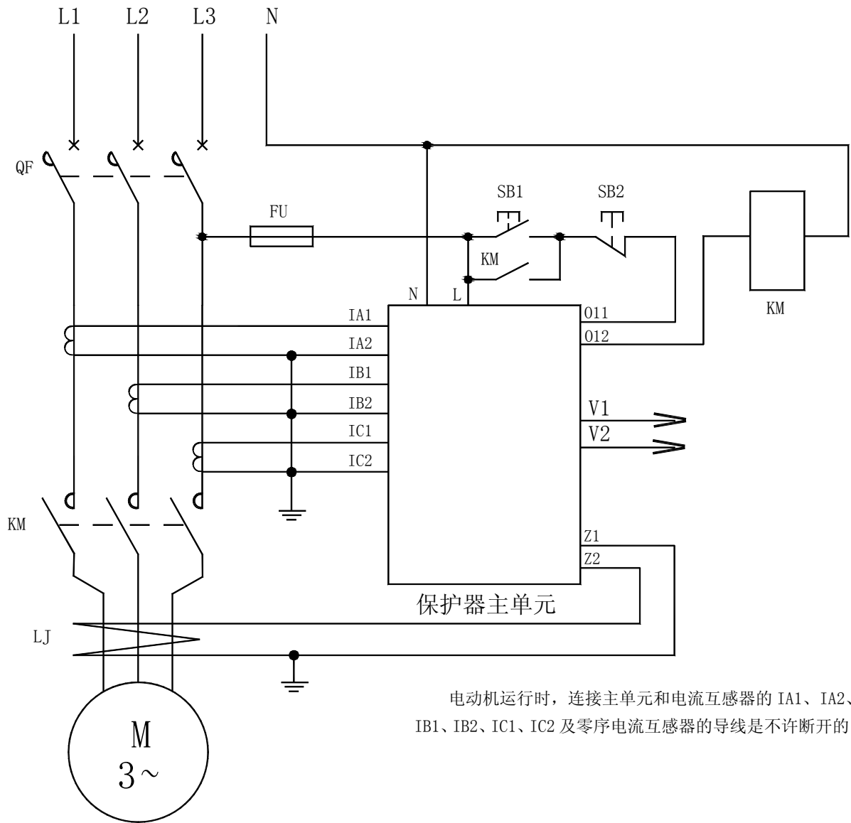
AMDG-X/F06□ 系列电动机保护器应用电气原理图
