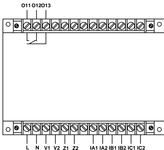
AMDG-X/F051 系列保护器主单元接线端子图
