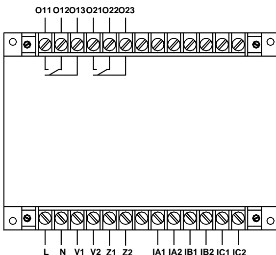
AMDG-X/F052 系列保护器主单元接线端子图
