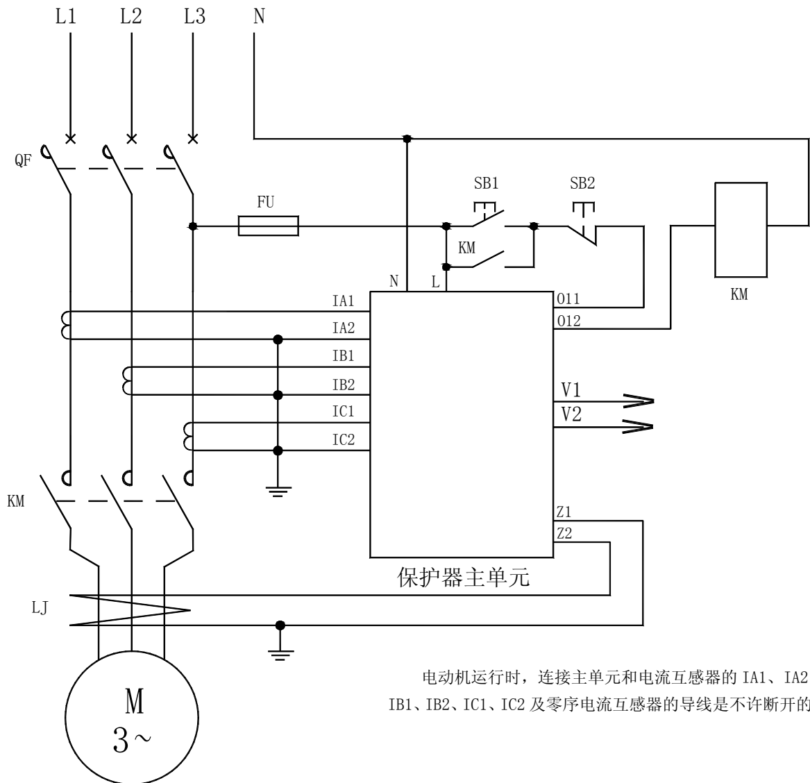
AMDG-X/F05□ 系列电动机保护器应用电气原理图
