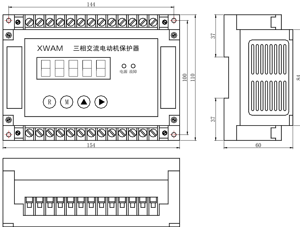
AMDG-X/F05□ 系列电动机保护器主单元外形及安装孔尺寸
