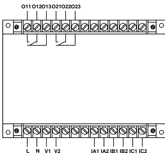
AMDG-X/F042 系列保护器主单元接线端子图
