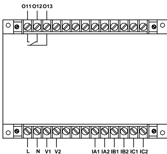
AMDG-X/F041 系列保护器主单元接线端子图
