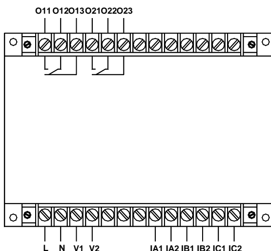
AMDG-X/F032 系列保护器主单元接线端子图
