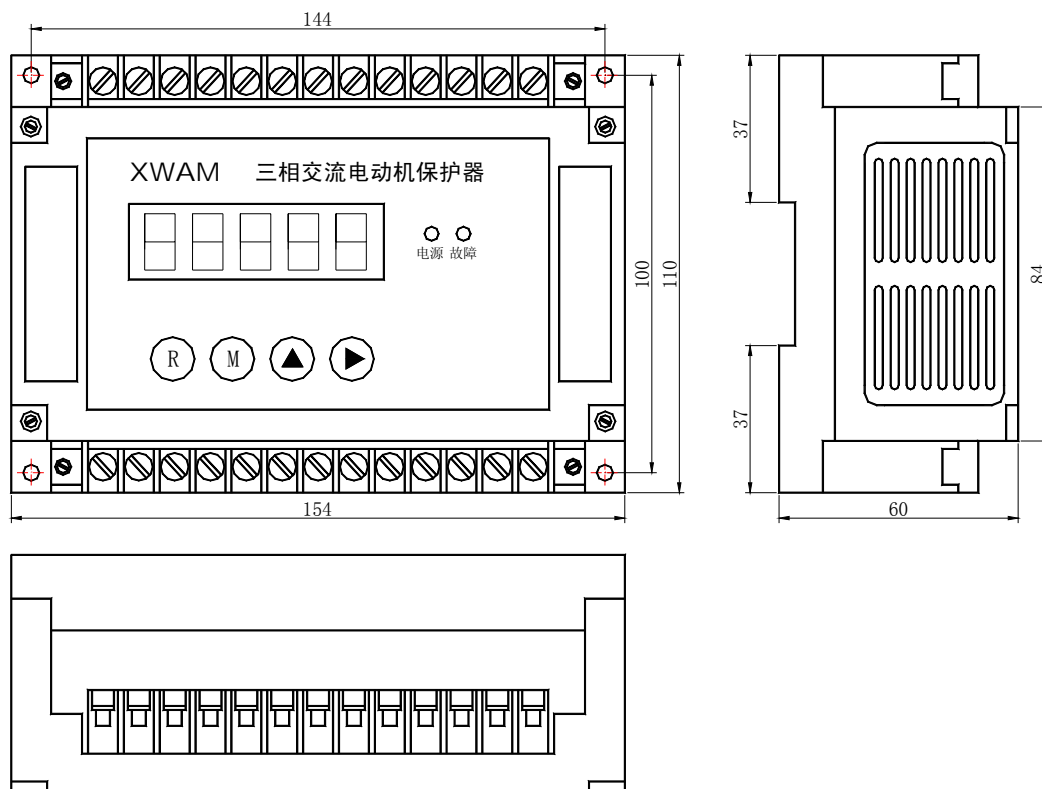
AMDG-X/F03□ 系列电动机保护器主单元外形及安装孔尺寸
