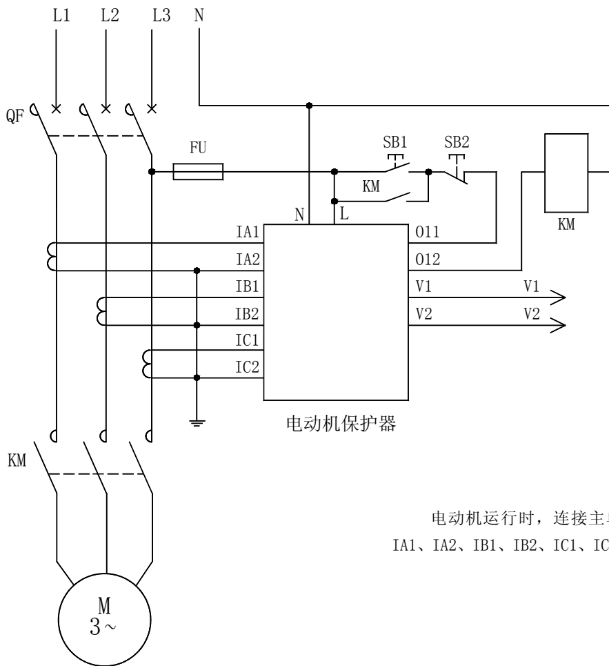
AMDG-X/F03□ 系列电动机保护器应用电气原理图
