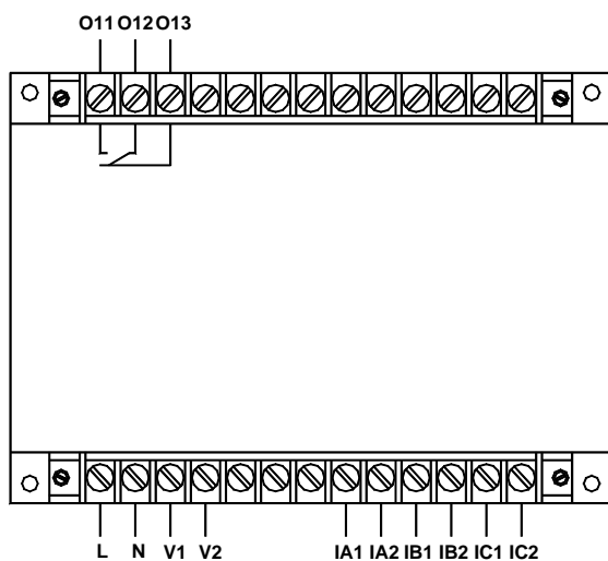
AMDG-X/F031 系列保护器主单元接线端子图
