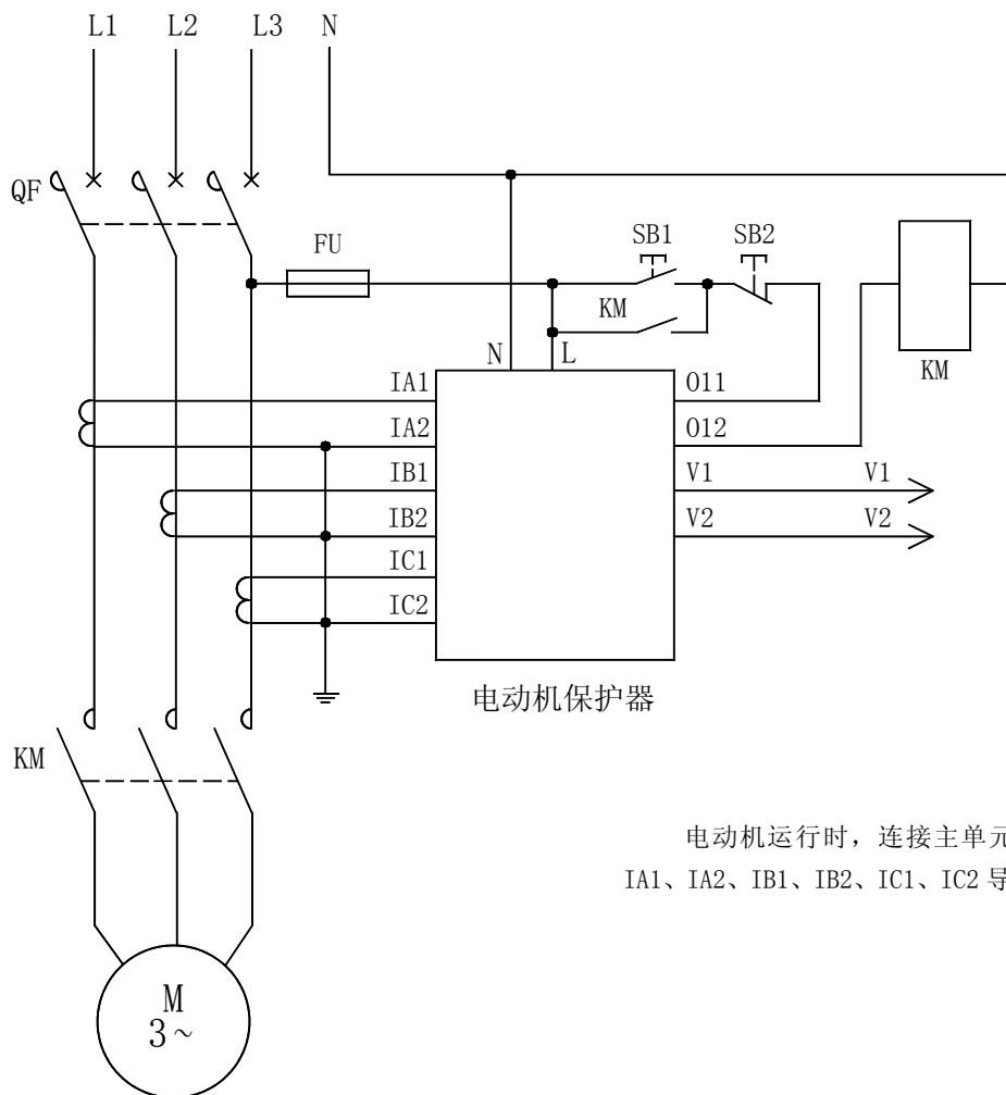
AMDG-X/F02□ 系列电动机保护器应用电气原理图
