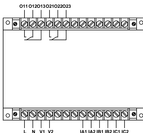
AMDG-X/F022 系列保护器主单元接线端子图
