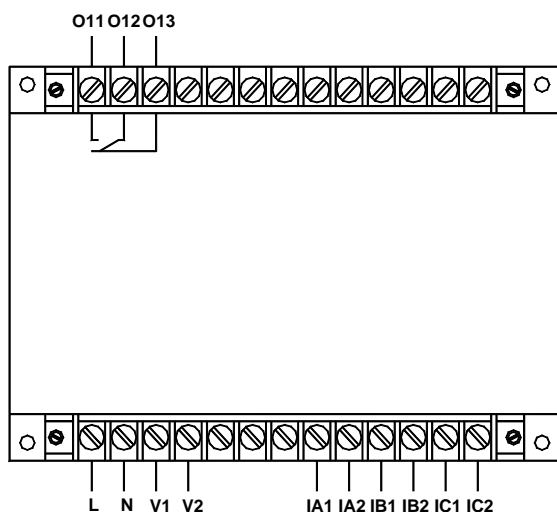
AMDG-X/F021 系列保护器主单元接线端子图
