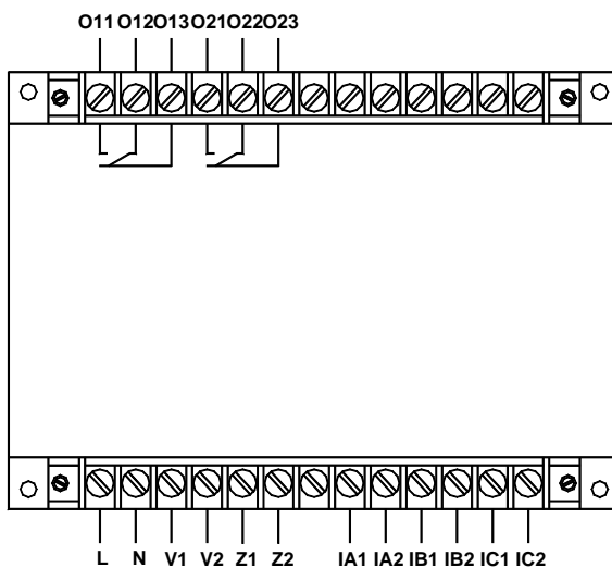
AMDG-X/F012 系列保护器主单元接线端子图
