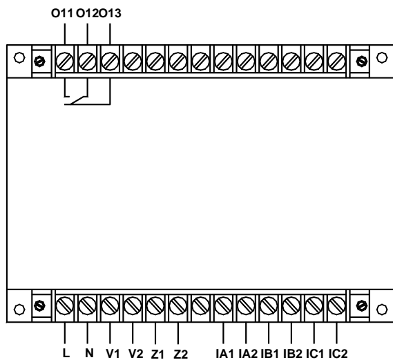
AMDG-X/F011 系列保护器主单元接线端子图
