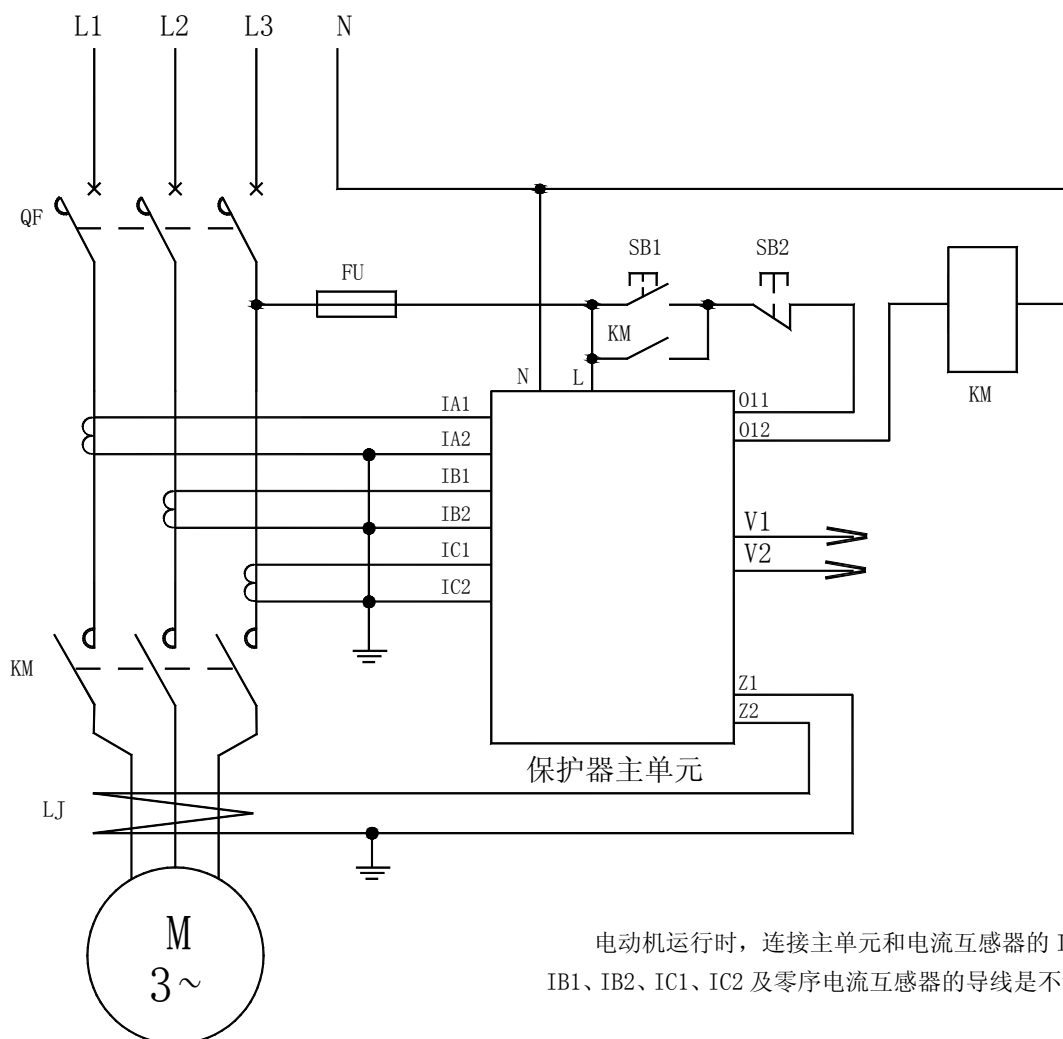
AMDG-X/F01□ 系列电动机保护器应用电气原理图
