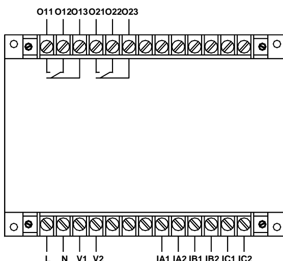
AMDG-X/F002 系列保护器主单元接线端子图
