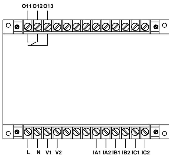
AMDG-X/F001 系列保护器主单元接线端子图
