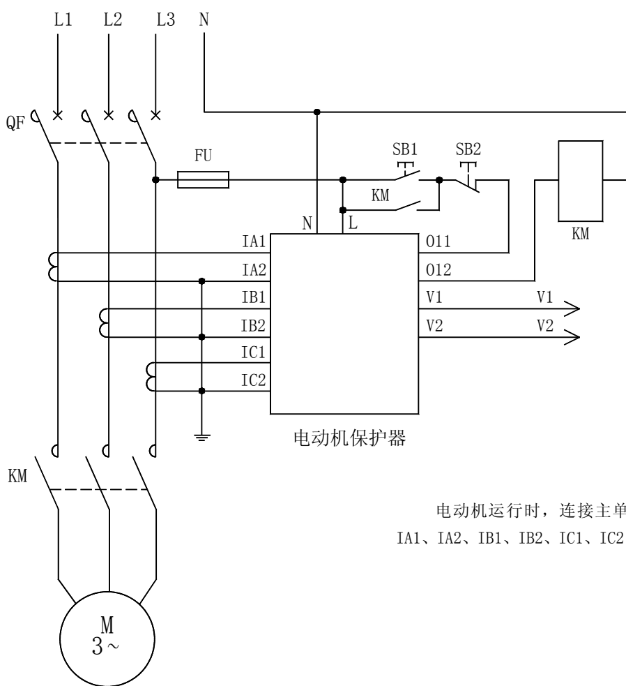
AMDG-X/F00□ 系列电动机保护器应用电气原理图
