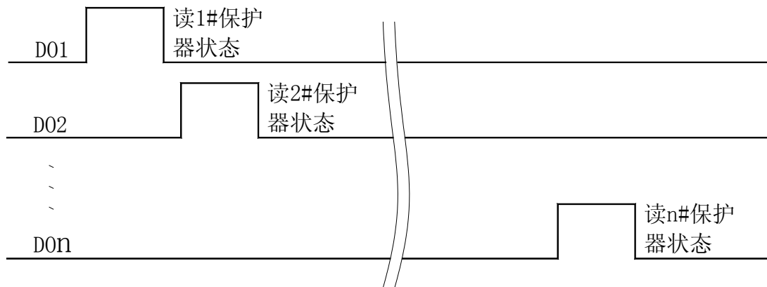
PLC 读取多台 AMDG-X/E851 系列电动机保护器时序图
