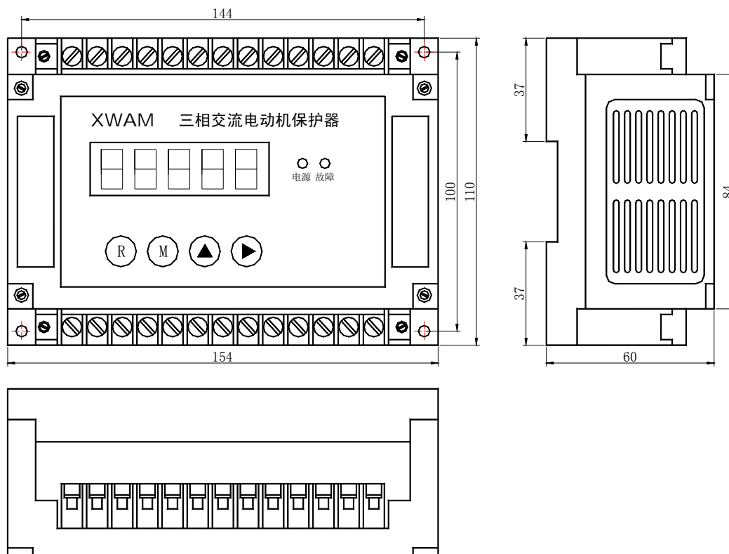
AMDG-X/E851 系列电动机保护器主单元外形及安装孔尺寸
