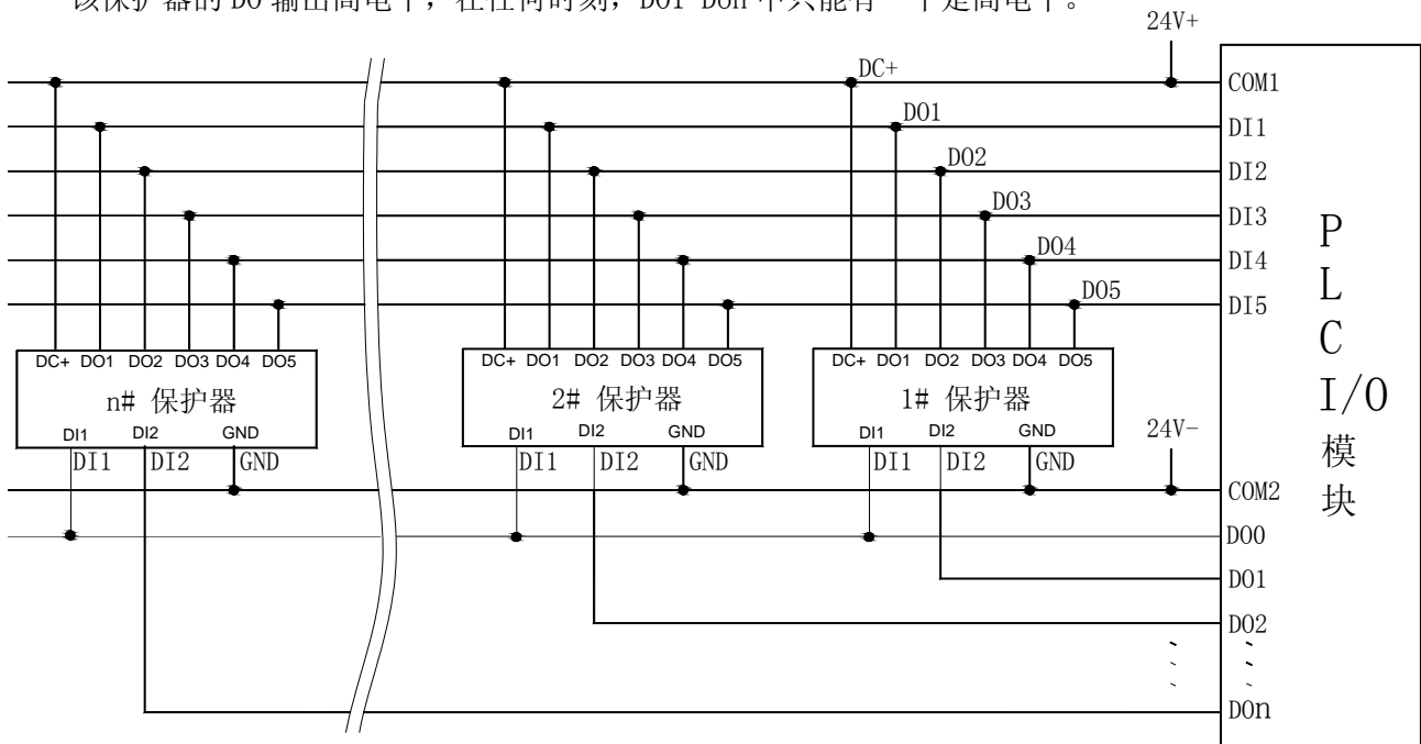
PLC 读取多台 AMDG-X/E851 系列电动机保护器电气原理图
