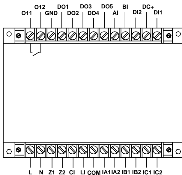
AMDG-X/E851 系列保护器主单元接线端子图
