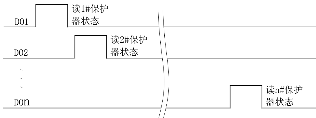
PLC 读取多台 AMDG-X/E821 系列电动机保护器时序图
