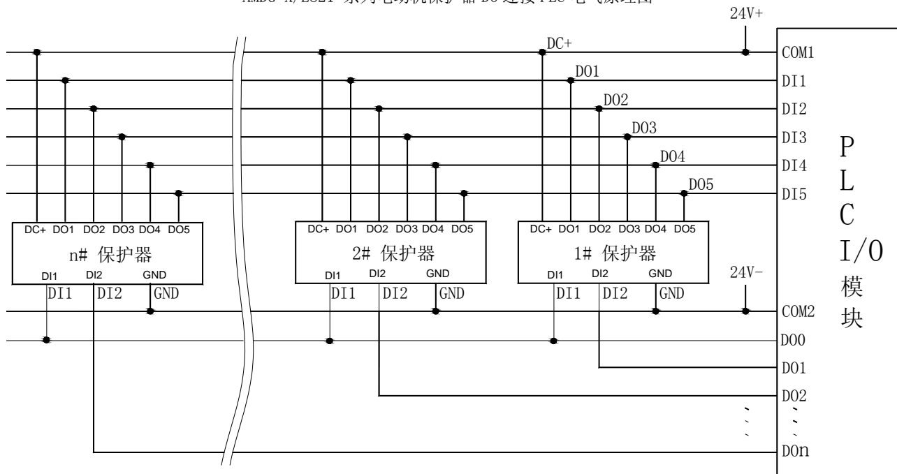
PLC 读取多台 AMDG-X/E821 系列电动机保护器电气原理图
