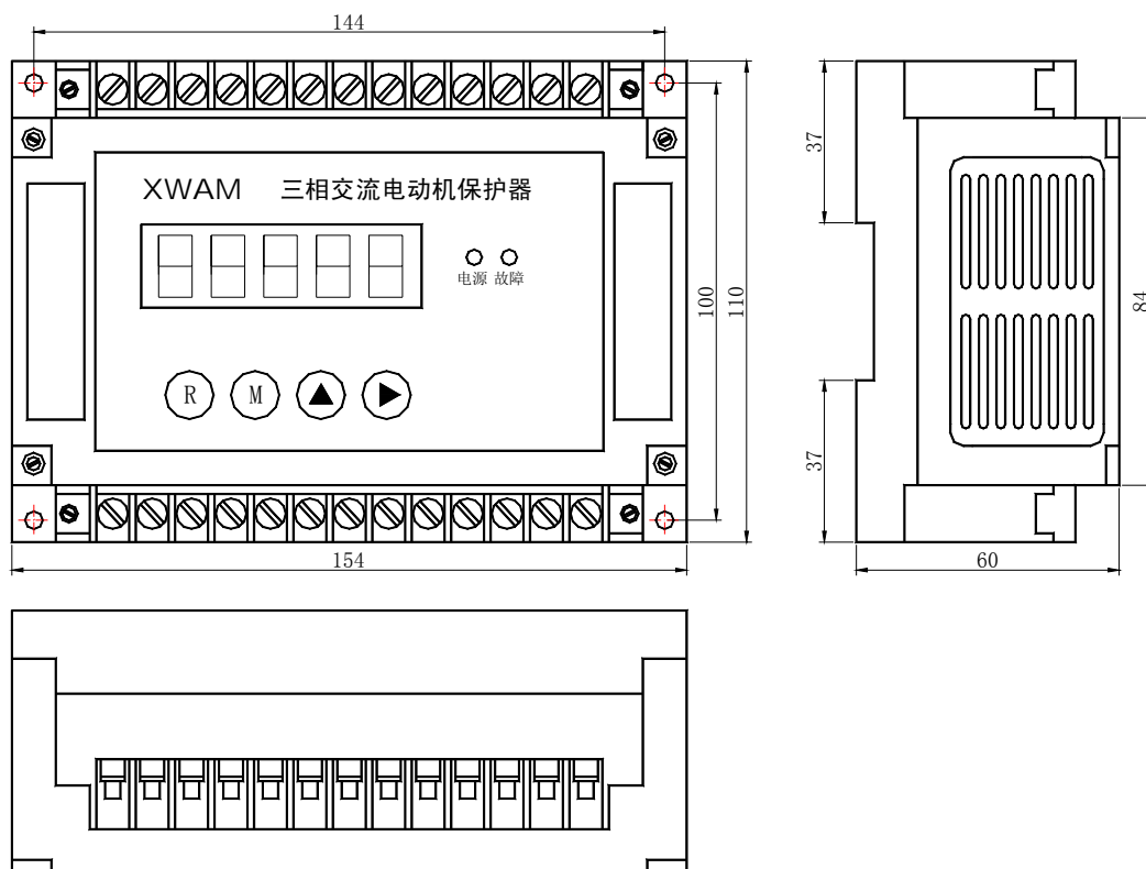
AMDG-X/E821 系列电动机保护器主单元外形及安装孔尺寸
