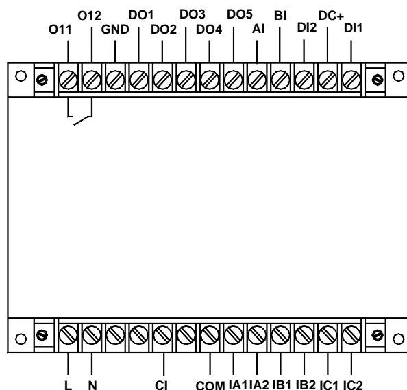
AMDG-X/E821 系列保护器主单元接线端子图
