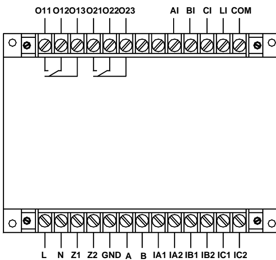
AMDG-X/E452 系列保护器主单元接线端子图
