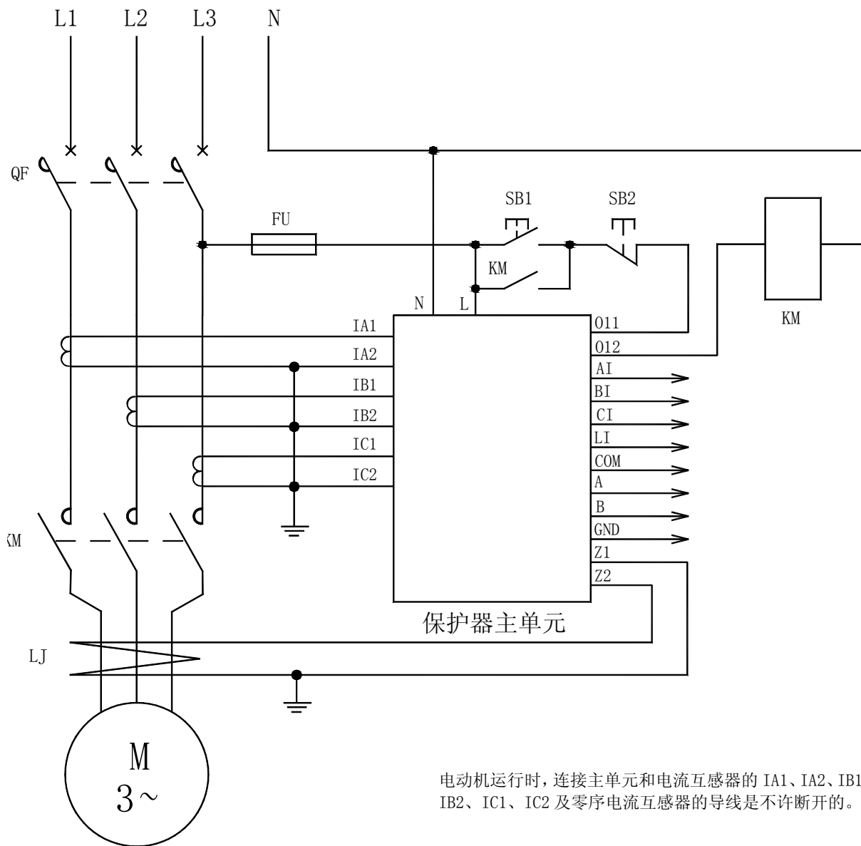
AMDG-X/E45□ 系列电动机保护器应用电气原理图
