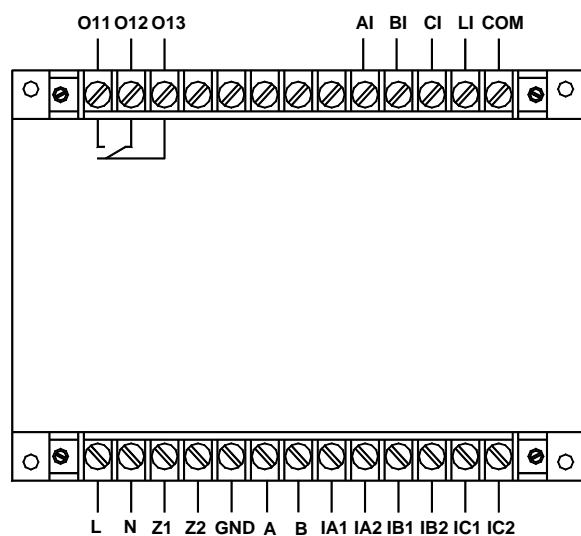
AMDG-X/E451 系列保护器主单元接线端子图
