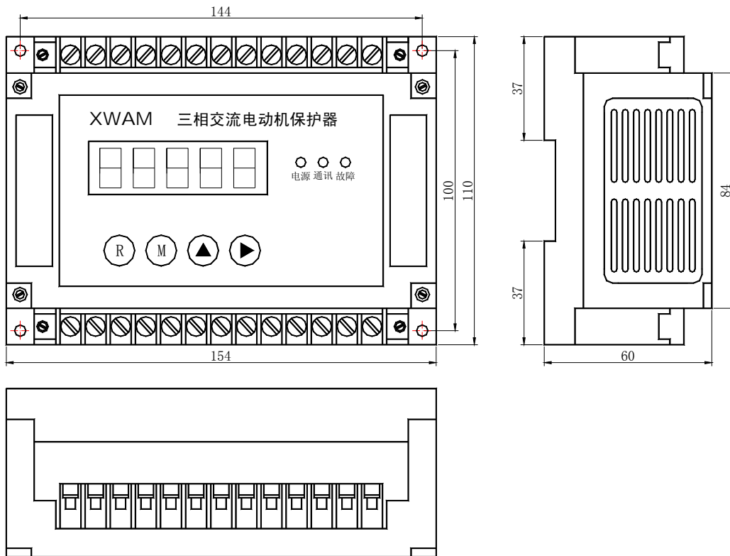
AMDG-X/E45□ 系列电动机保护器主单元外形及安装孔尺寸
